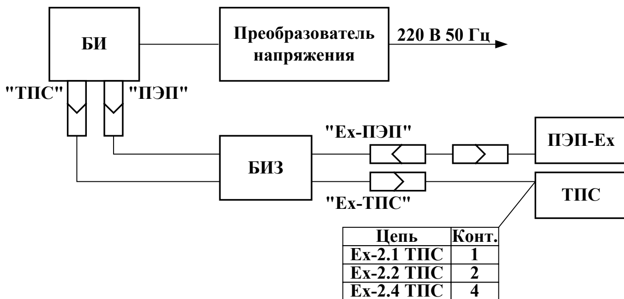
Рис.Б.2. Схема подключения УР-Ех / РСЛ-Ех с использованием ТПС.
