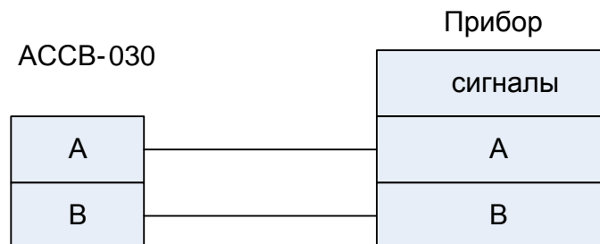
Рис.4. Подключение прибора по интерфейсу RS-485.
