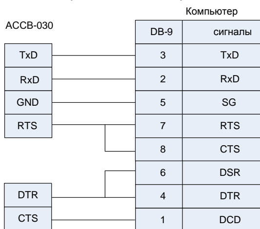
Рис.11. Схема подключения АССВ-030 к компьютеру в качестве универсального модема.
