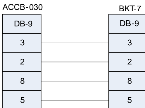
Рис.6. Подключение ACCB-030 к ВКТ-7.
