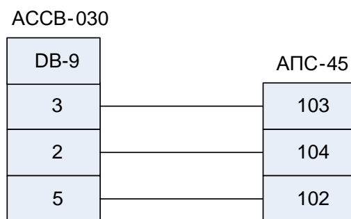
Рис.5. Подключение АССВ-030 к АПС-45.
