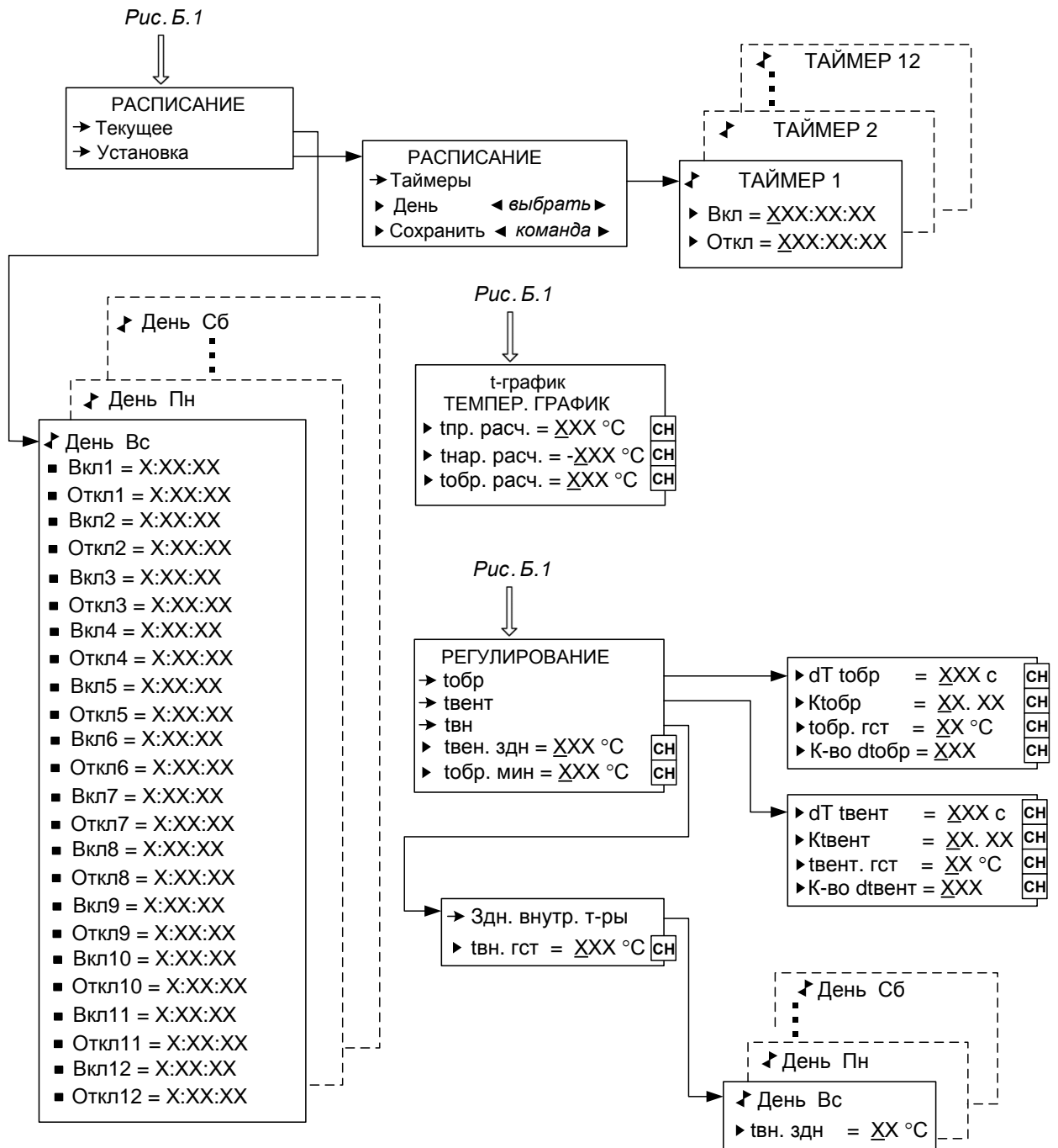
Рис.Б.2. Меню Расписание, t-график и Регулирование.
