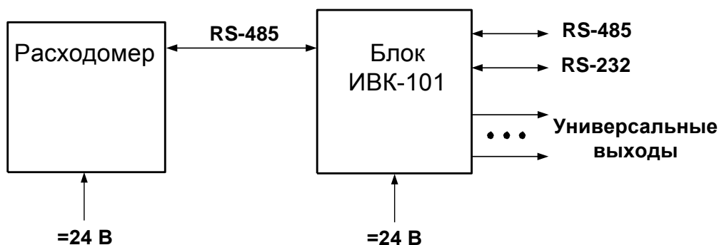
Рис.4. Система сбора данных и выносной индикации на базе комплекса «ВЗЛЕТ ИВК» исполнения ИВК-101 для одного расходомера.
