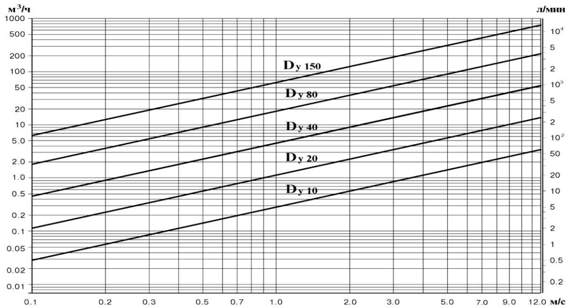
Рис.5. График зависимости расхода жидкости от скорости потока для различных значений D_\gamma .
