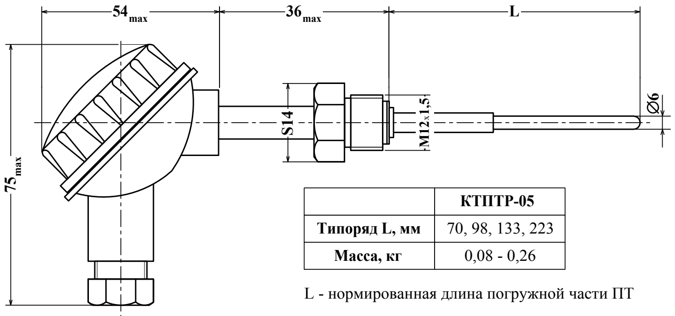
Рис. А.4. Внешний вид ПТ типа КПТПР-05.
