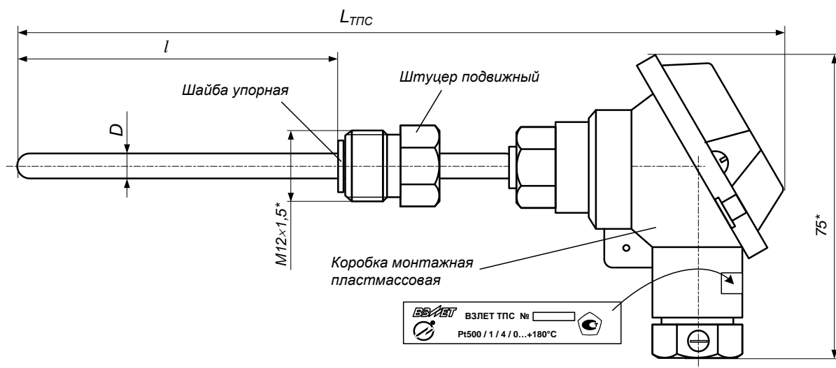
а) ТПС с подвижным штуцером (винчиваемый)
