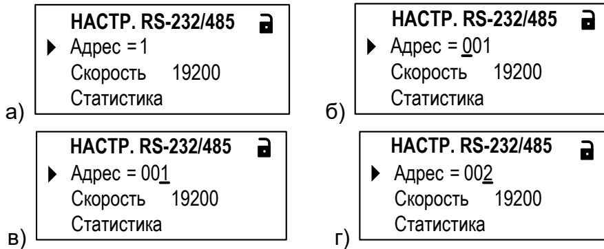
Рис.11. Вид окна индикации при вводе значения параметра поразрядно.
