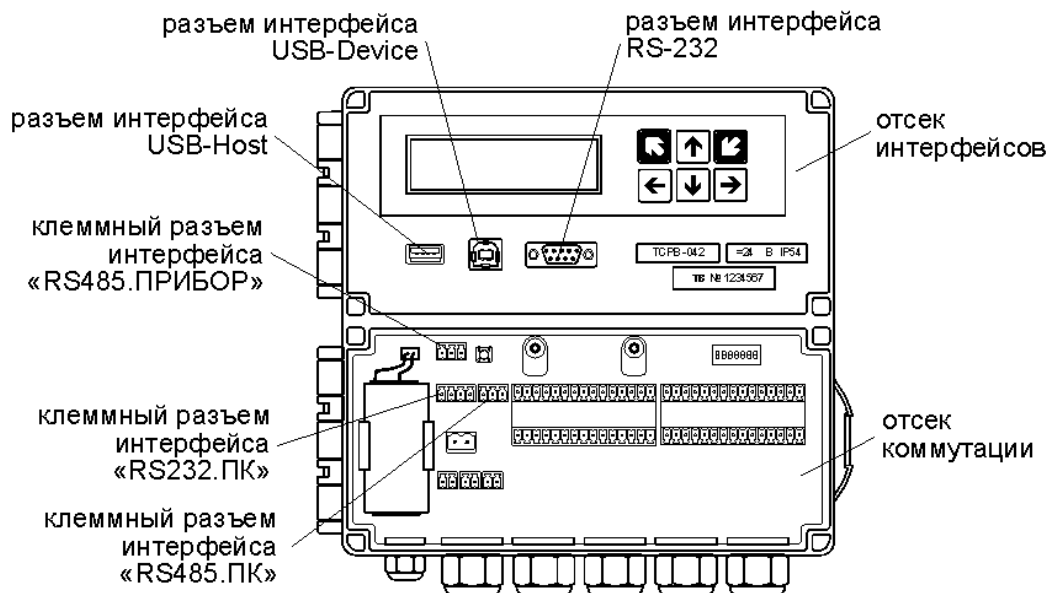
Рис.14. Размещение интерфейсных разъемов тепловычислителя.
