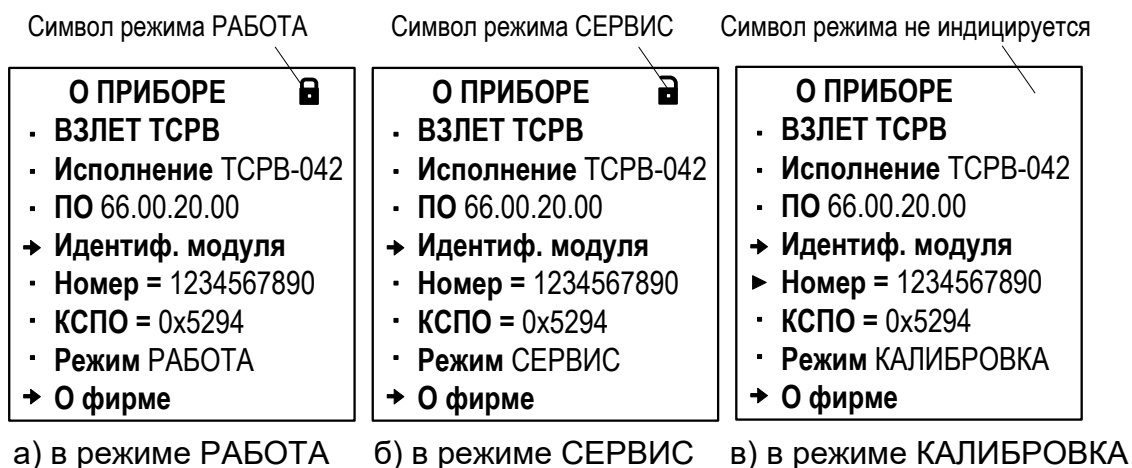
Рис.6. Вид окон индикации «О ПРИБОРЕ» в различных режимах.
