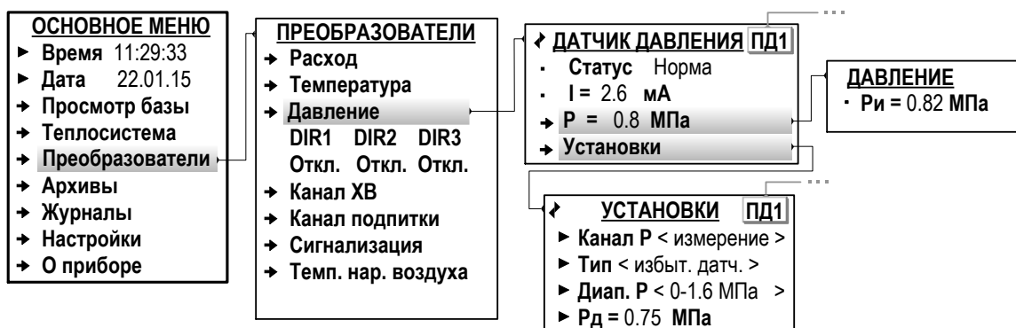
Рис.31. Вид меню настройки ПД (режим СЕРВИС).
