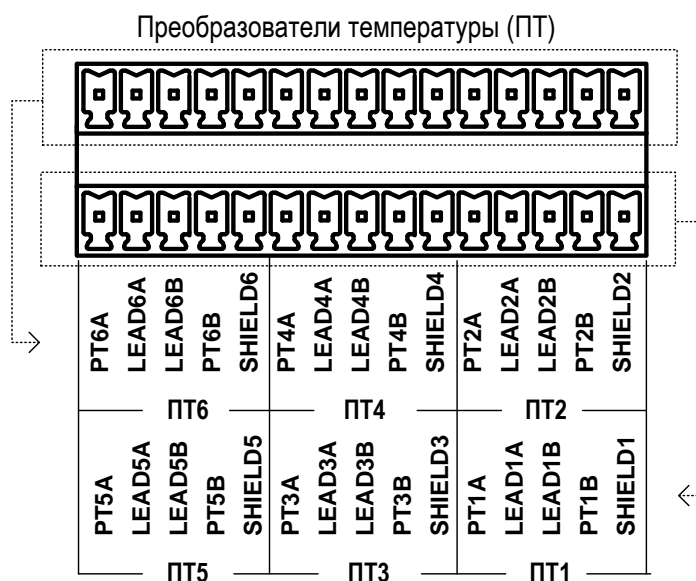
Рис.28. Обозначение коммутационных элементов подключения ПТ.
