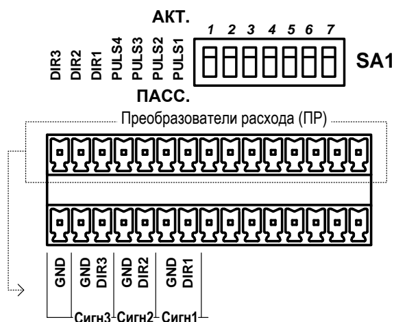
Рис.26. Маркировка коммутационных элементов подключения входов «Сигнализация».
