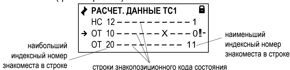
Рис.7. Отображение символов в знакопозиционном коде состояния.
