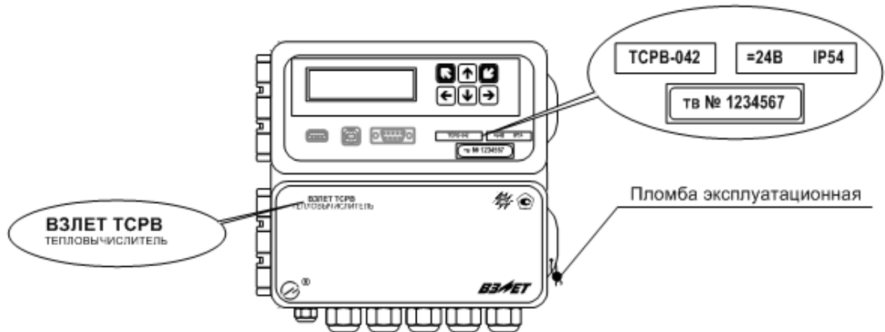
Рис.3. Вид и размещение маркировки и возможных мест пломбирования корпуса ТВ.
