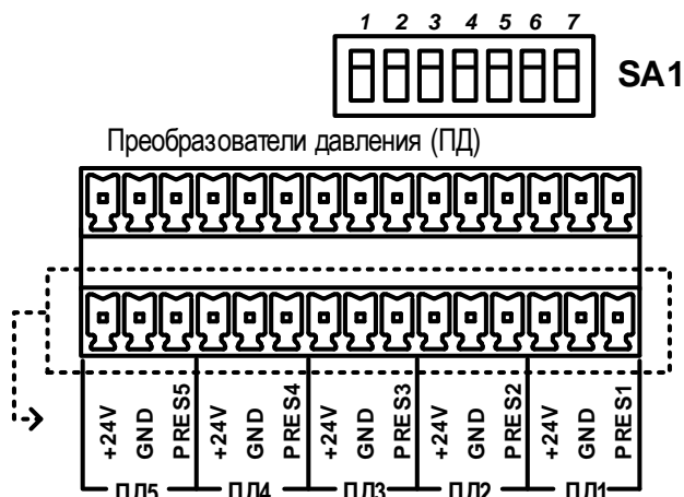
Рис.30. Обозначение коммутационных элементов подключения ПД.
