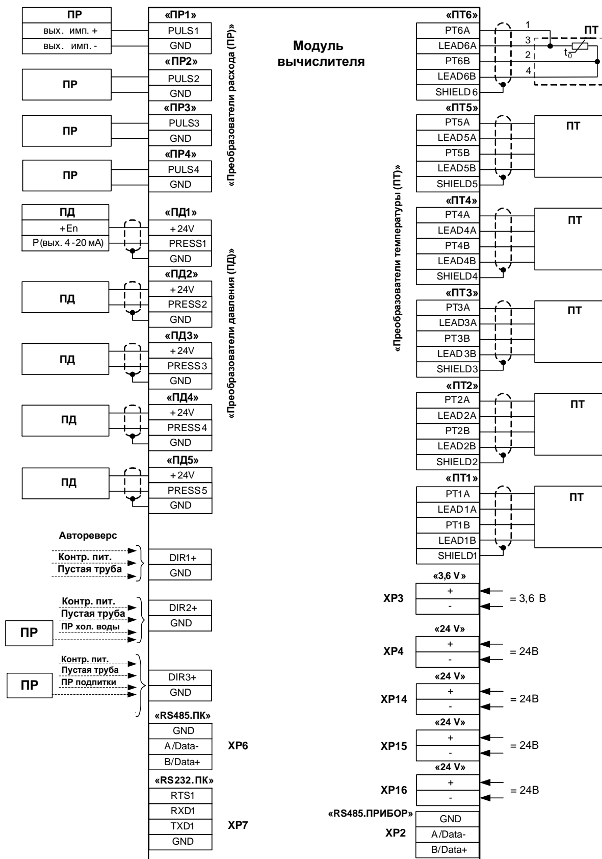
Рис.Б.1. Схема подключений модуля вычислителя.
