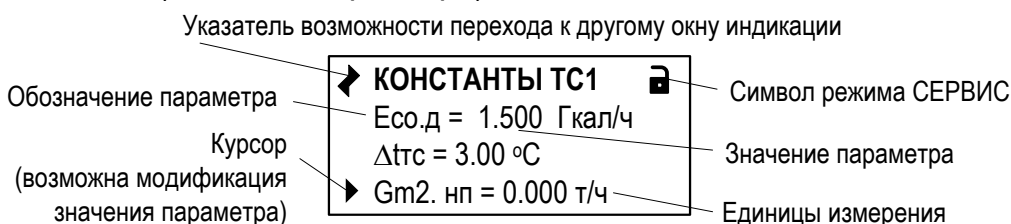
Рис.8. Вид одного из окон индикации многооконного меню.
