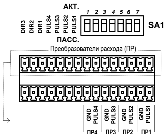
Рис.22. Маркировка коммутационных элементов подключения ПР.
