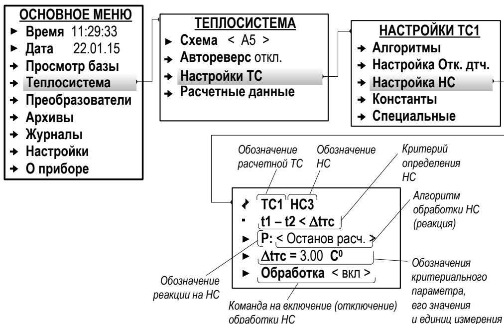
Рис.37. Вид меню настройки обработки НС (режим СЕРВИС).
