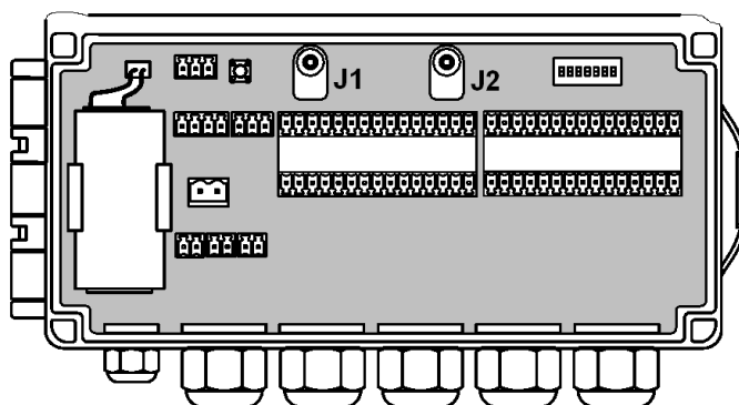
Рис.4. Расположение контактных пар J1 и J2 в отсеке коммутации.
