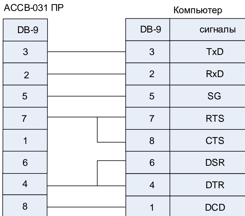
Рис.11. Схема подключения АССВ-030 ПР к компьютеру в качестве универсального модема.
