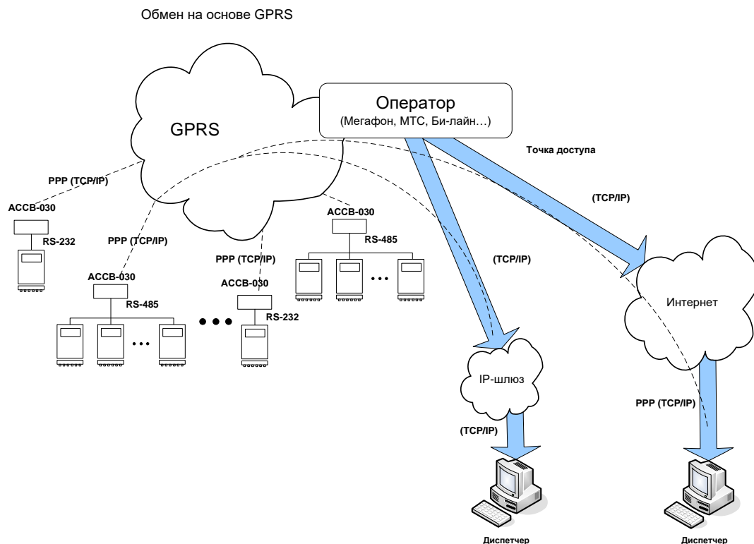
Рис.2. Схема организации обмена на основе GPRS.
