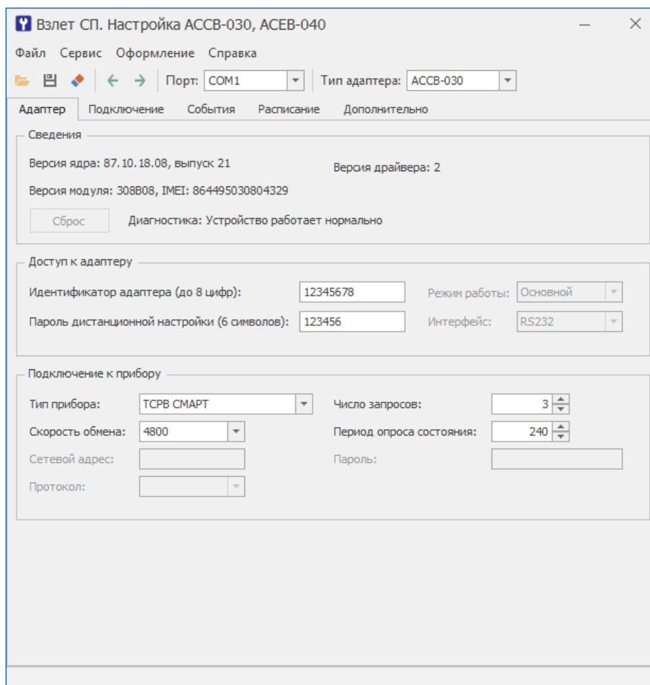
Рис.5. Основное окно программы «Взлет СП. Настройка АССВ-030, АСЕВ-040».
