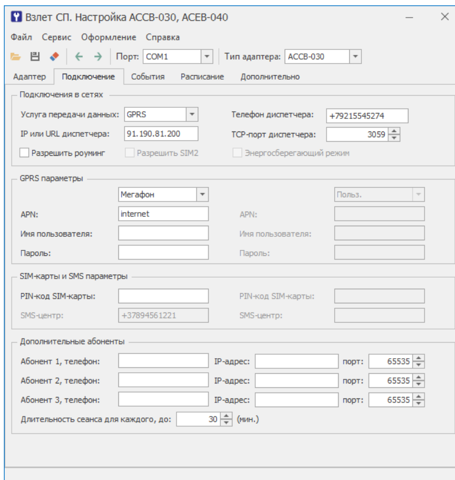
Рис.7. Вкладка «Подключение» программы «Взлет СП. Настройка ACCB-030, ACEB-040».
