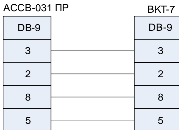
Рис.15. Подключение прибора к ВКТ-7.
