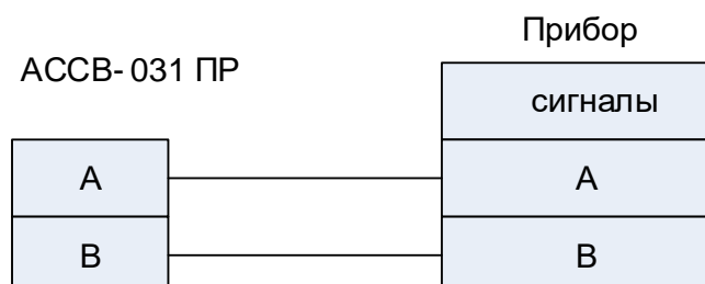
Рис.13. Подключение прибора по интерфейсу RS-485.
