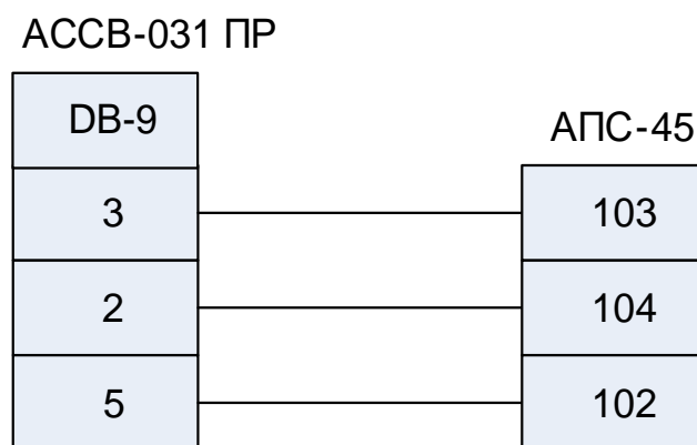
Рис.14. Подключение прибора к адаптеру АПС-45.
