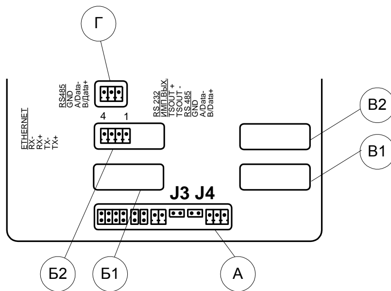
Рис.В.4. Маркировка коммутационных элементов модуля интерфейса Ethernet.
