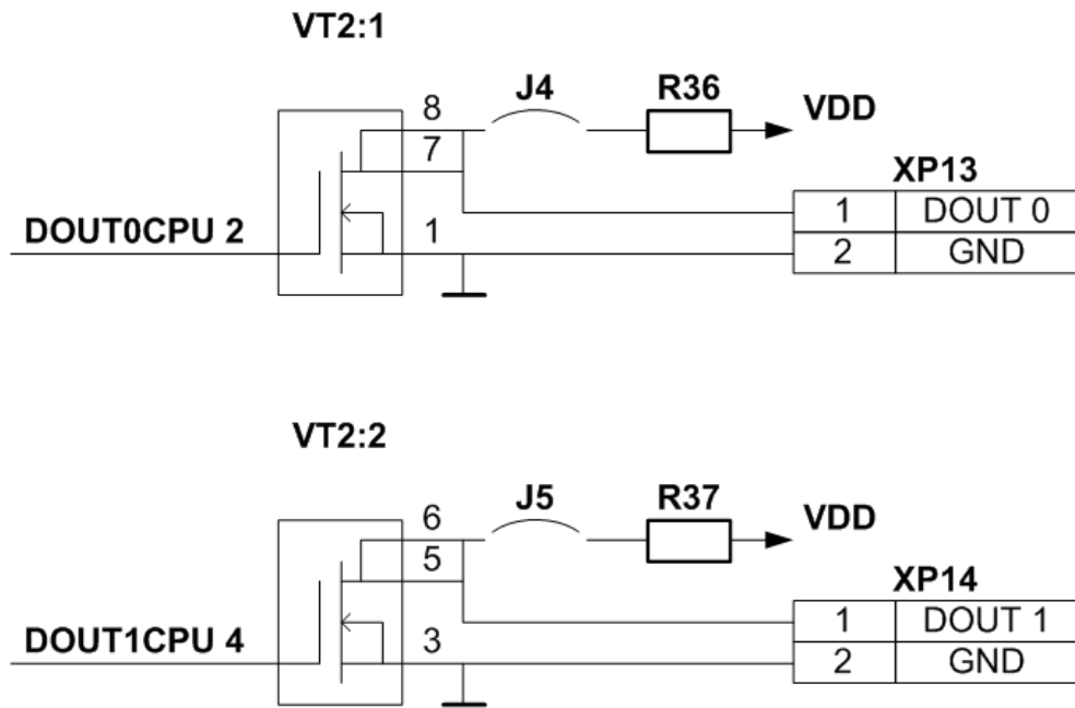
Рис.Б.3. Схема окончных каскадов дискретных выходов модуля обработки данных ИВК исполнения ИВК-102.
