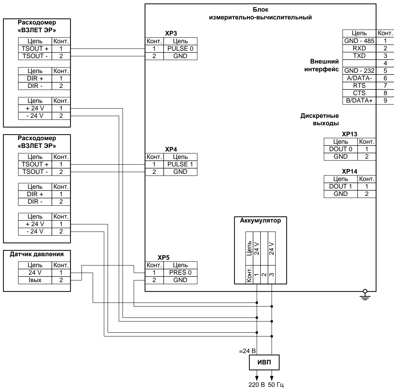
Рис.Б.2. Схема подключения к ИВК исполнения ИВК-102 двух расходомеров и датчика давления с питанием от ИВП комплекса.
