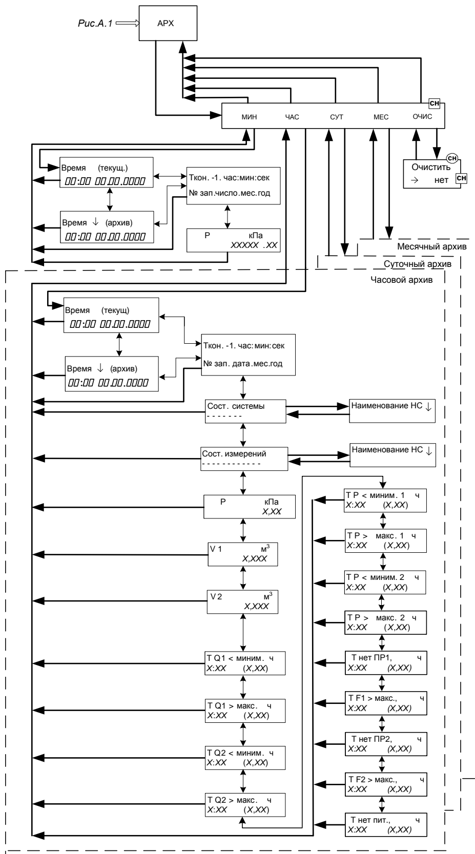
Рис.А.5. Меню «APX».
