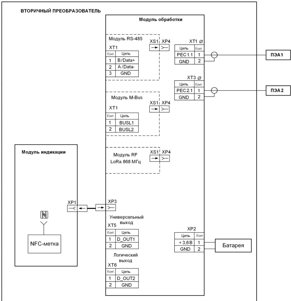
Рис.Б.1. Схема соединений расходомера УПСВ-310.
