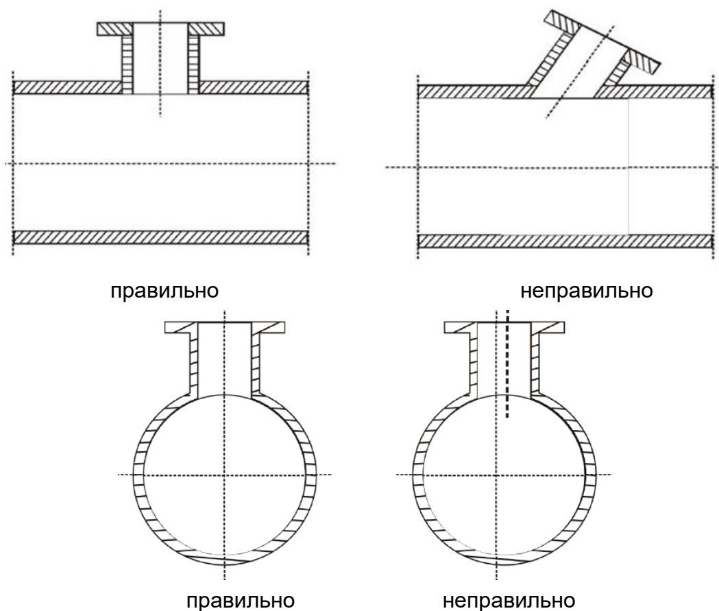
Рис.2. Правильное монтажное положение соединительного основания
