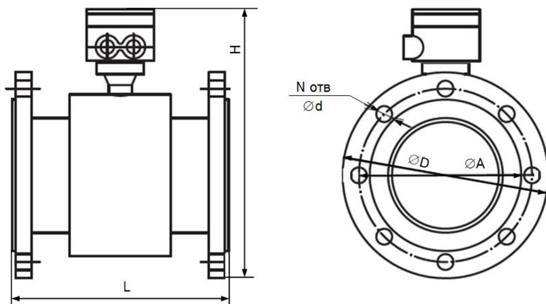
Рис.А.2. Первичный преобразователь расходомера EM470 разнесенного фланцевого исполнения
