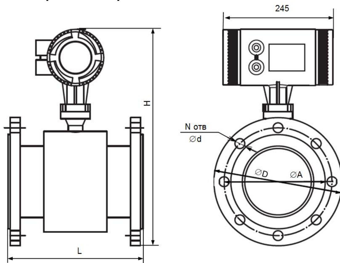
Рис.А.1. Расходомер EM470 компактного фланцевого исполнения
