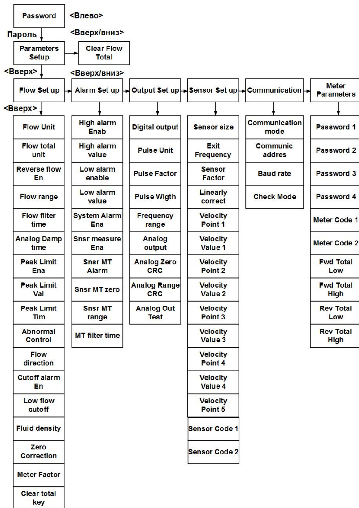
Рис.Б.1. Структура меню расходомера
