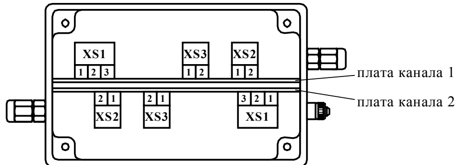
Рис. В.1. Вид адаптера токового выхода.
