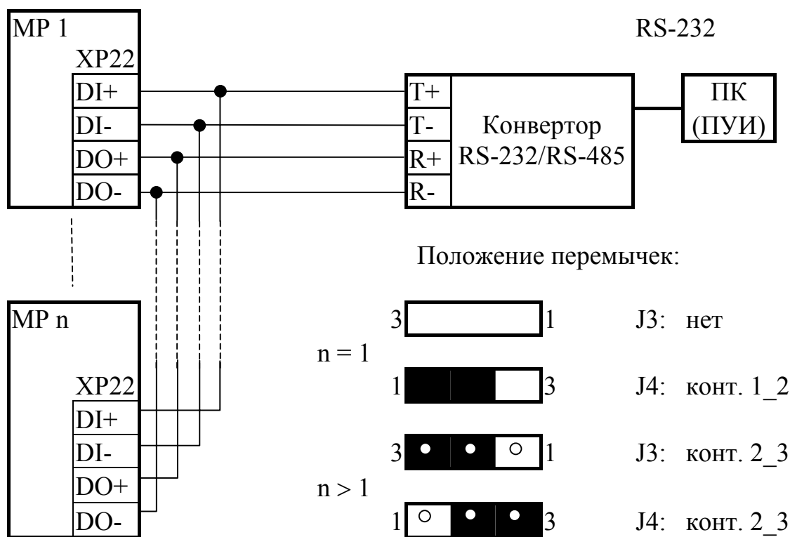
а) при четырехпроводной линии связи
