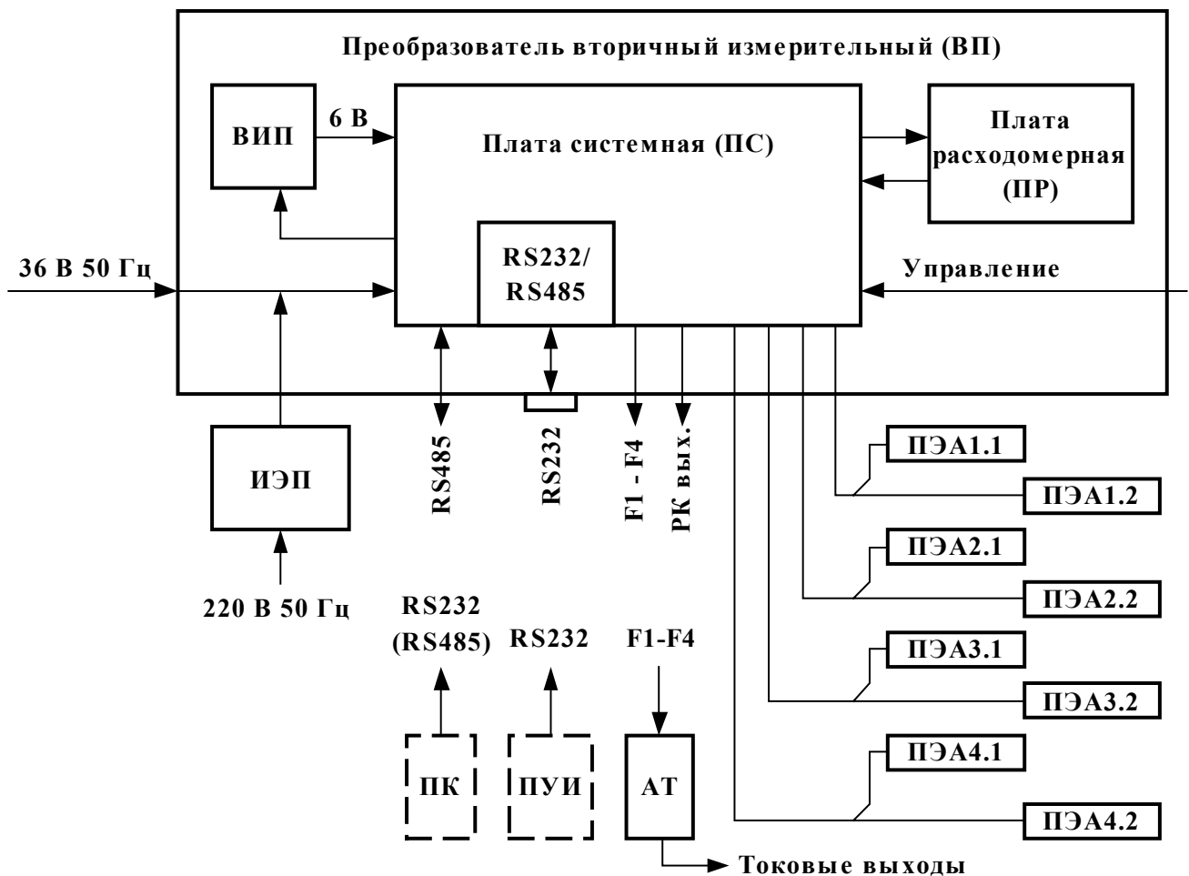
Рис. 1. Структурная схема расходомера.
