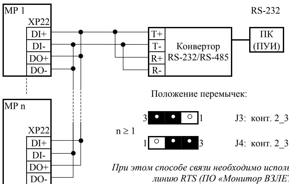
б) при двухпроводной линии связи
