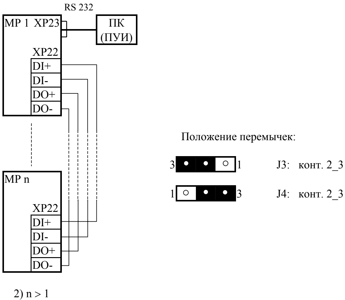
Рис. Б.6. Схема подключения ПК (ПУИ) к расходомеру с использованием встроенного конвертера RS-232/RS-485.
