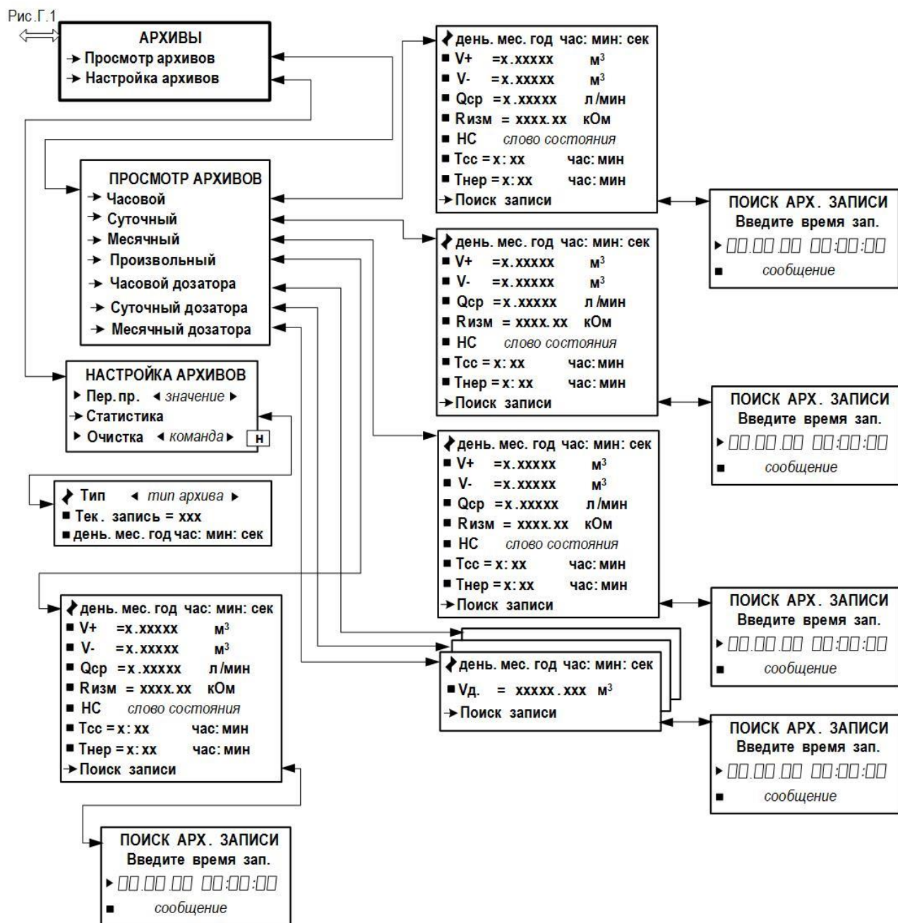
Рис.Г.7. Меню «АРХИВЫ».
