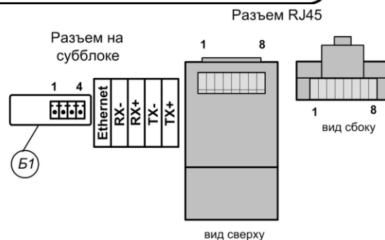
Рис.А.4. Обозначения коммутационных элементов на субблоке вычислителя ТЭР, расположенные на тыльной стороне крышки прибора.
