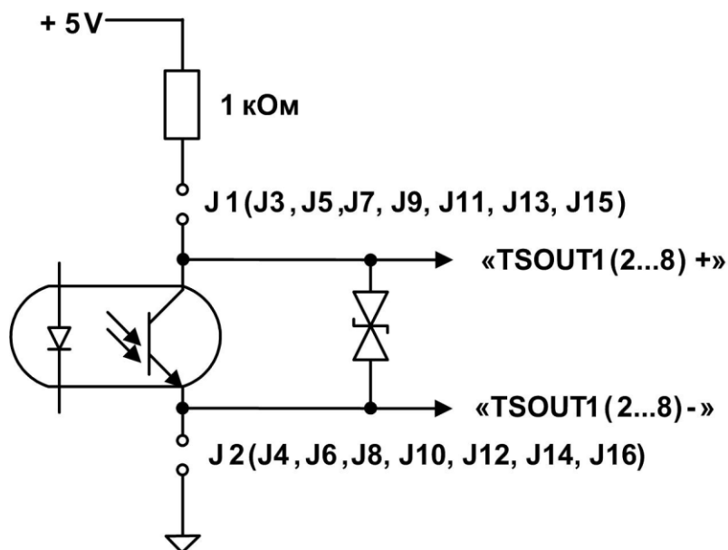
Рис.Б.1. Схема окончного каскада универсальных выходов комплекса.
