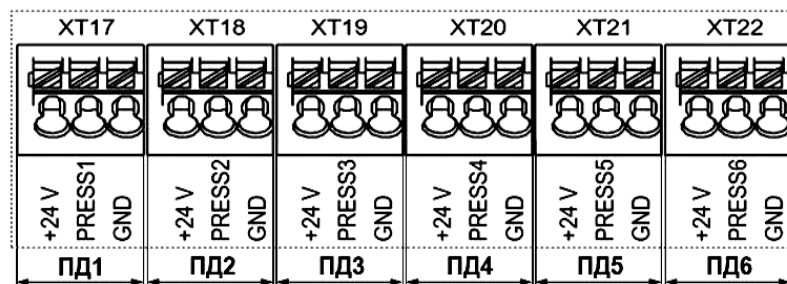
Рис.В.2. Коммутационные элементы подключения ПД1...ПД6.
