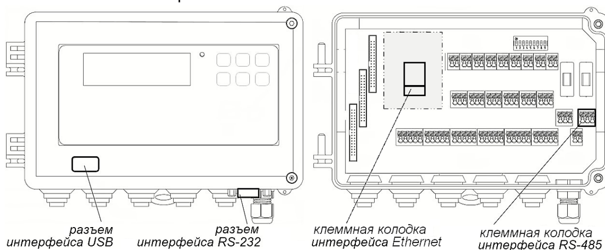
Рис.11. Размещение интерфейсных разъемов тепловычислителя.
