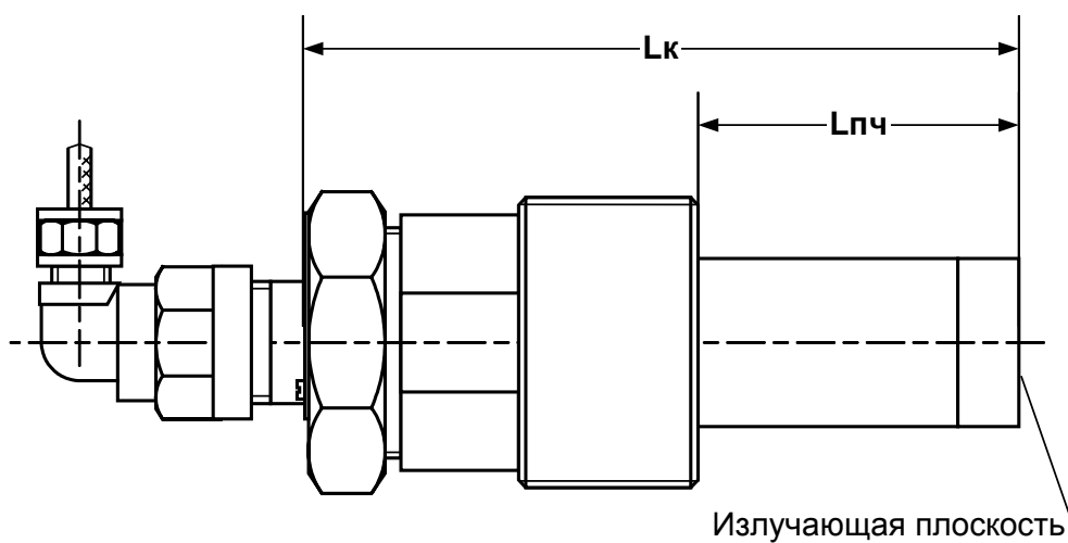
Рис. 13. Вид врезного ПЭА.
