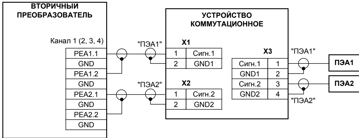
Рис. Б.2. Схема подключения пары ПЭА при несимметричной схеме связи с использованием устройства коммутационного.
