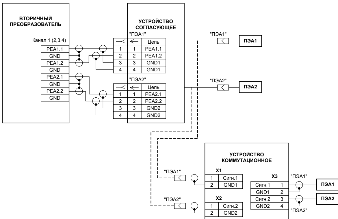
Рис. Б.3. Схема подключения пары ПЭА при симметричной схеме связи с использованием устройства коммутационного.
