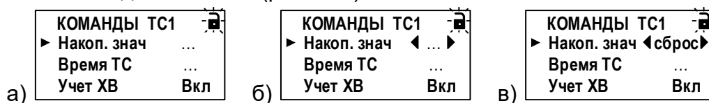
Рис.10. Вид окна индикации команды сброса накопленных значений.
