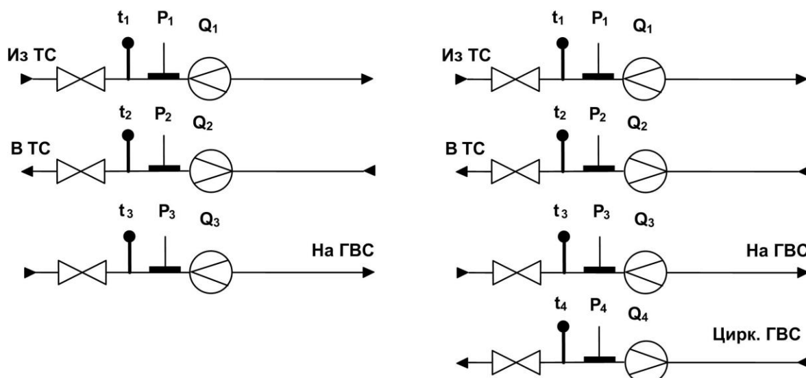
Рис.17. Схемы теплоснабжения с подпиткой из различных трубопроводов
