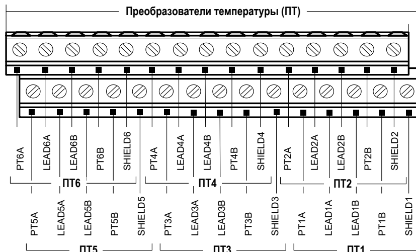
Рис.28. Обозначение коммутационных элементов подключения ПТ.
