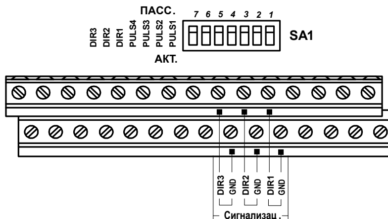
Рис.26. Маркировка коммутационных элементов подключения входов «Сигнализация».
