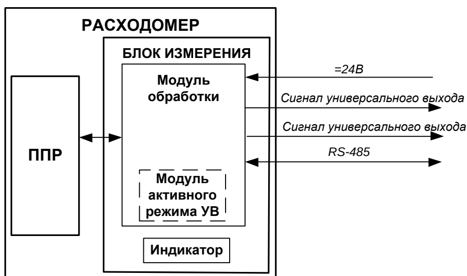
б) исполнение ППД-213 с модулем активного режима универсальных выходов
