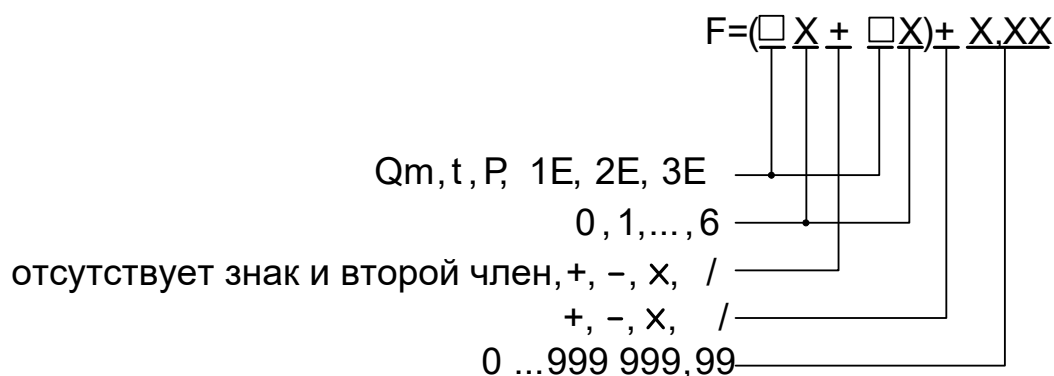
Рис.5. Структура и возможные значения членов формулы для частотно-импульсного режима работы.
