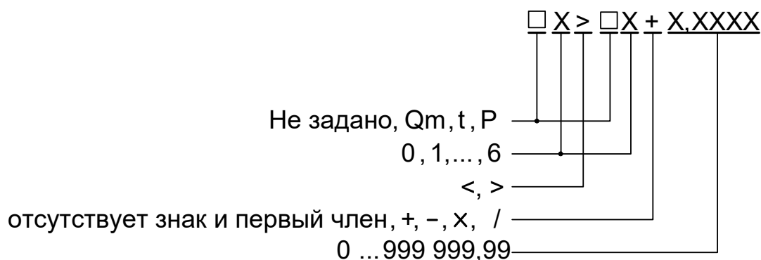
Рис.3. Структура и возможные значения членов формулы критериев оценки наличия нештатных ситуаций HC1-HC3.
