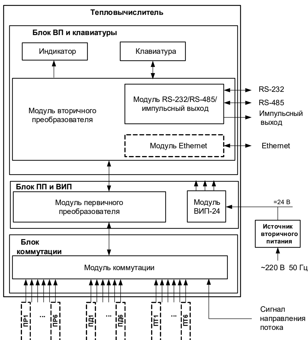
Рис.1. Структурная схема тепловычислителя.
