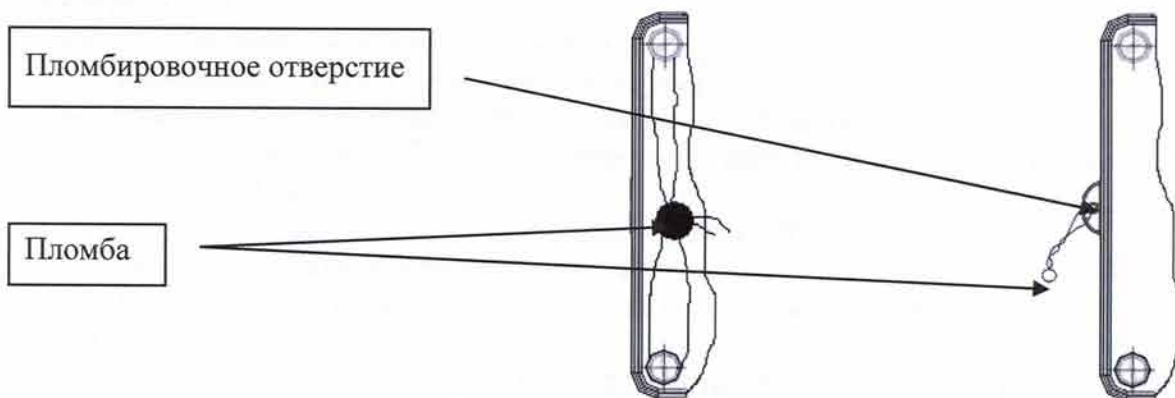
Рисунок. 2 - Схема пломбировки теплосчетчиков - регистраторов «ВЗЛЕТ ТСП-М»
