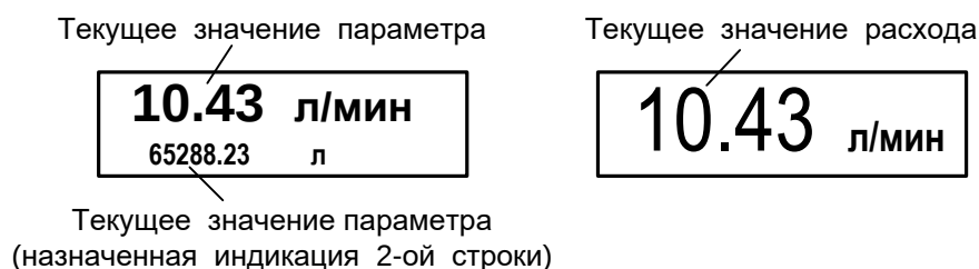
Рис.5. Вид окон укрупненной индикации измеряемого параметра.
