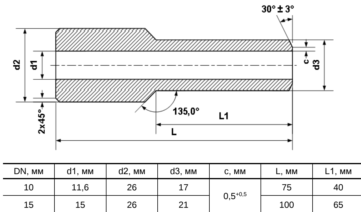
Рис.В.3. Вид и размеры переходных патрубков DN10, DN15.
