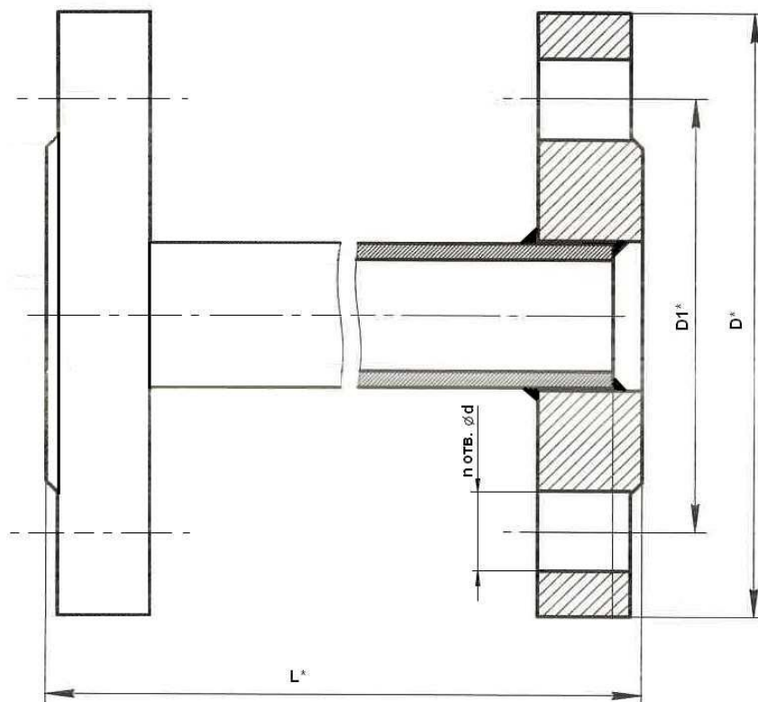
Рис.Б.3. Вид габаритного имитатора фланцованных ППР для монтажа с защитными кольцами.
