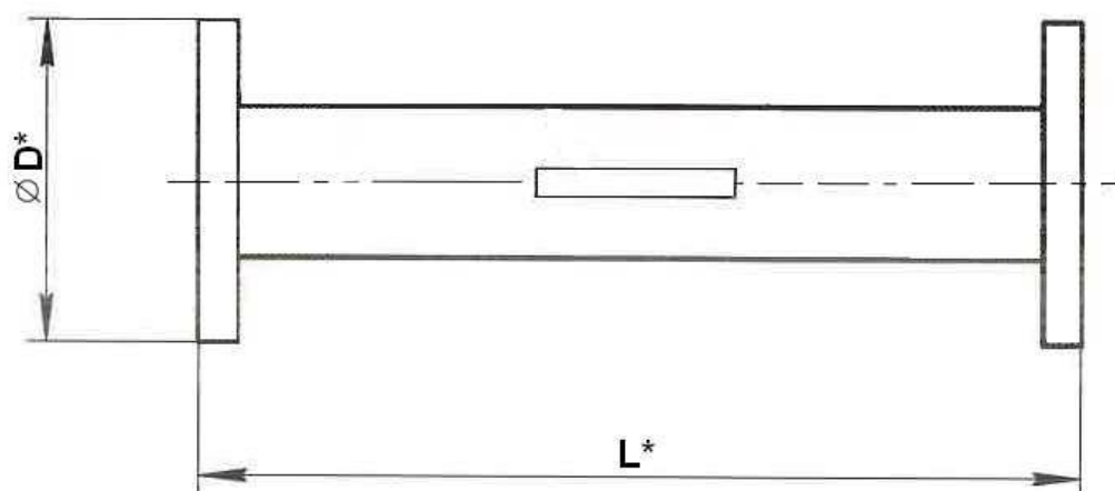
Рис.Б.1. Вид габаритного имитатора ППР типа «сэндвич» для монтажа с защитными кольцами.
