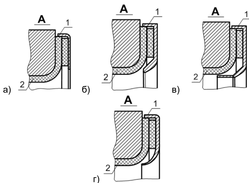
Рис. А.4. Вид ППР с защитными кольцами разных исполнений:
