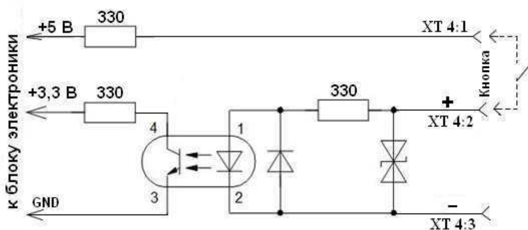
Рис.Г.3. Схема входа управления дозированием БИ.
