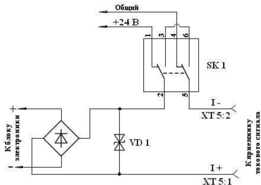
Рис.Г.2. Схема токового выхода расходомера (активный режим).
