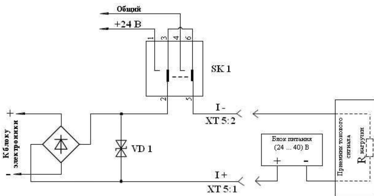
Рис.Г.3. Схема токового выхода расходомера (пассивный режим).
