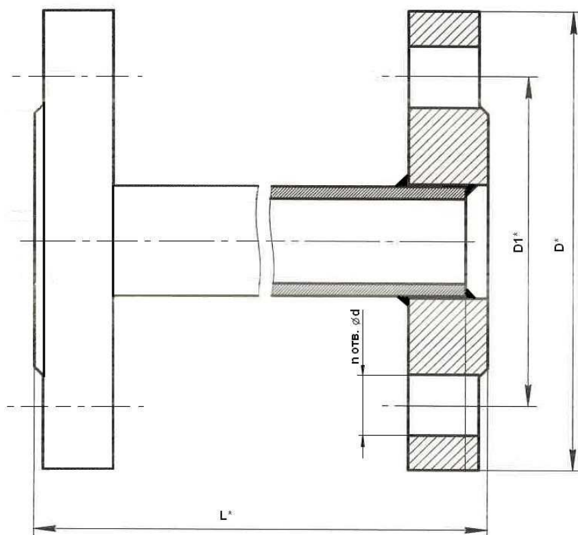
Рис.Б.4. Вид габаритного имитатора фланцованных ППР для монтажа без защитных колец.
