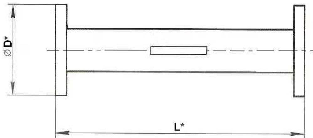
Рис.Б.2. Вид габаритного имитатора ППР типа «сэндвич» для монтажа без защитных колец.
