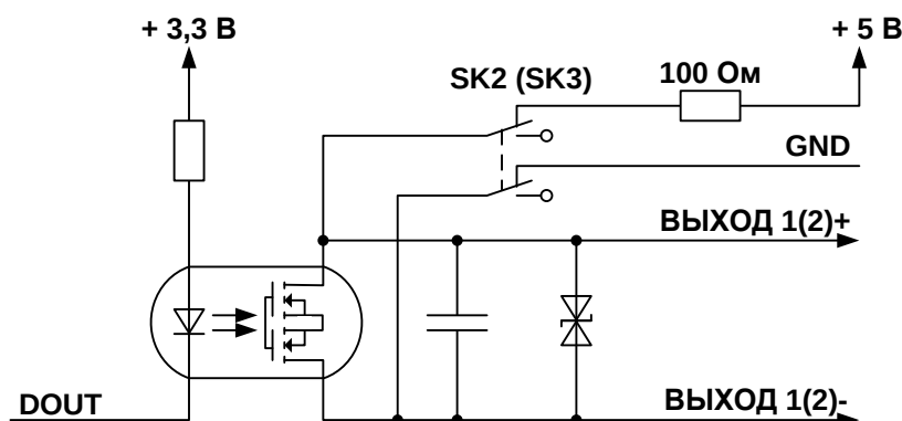
Рис.Г.1. Схема оконечного каскада универсальных выходов.
