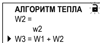
Рис.11. Вид окна индикации расчетной формулы, расположенной в одной строке с обозначением параметра.
