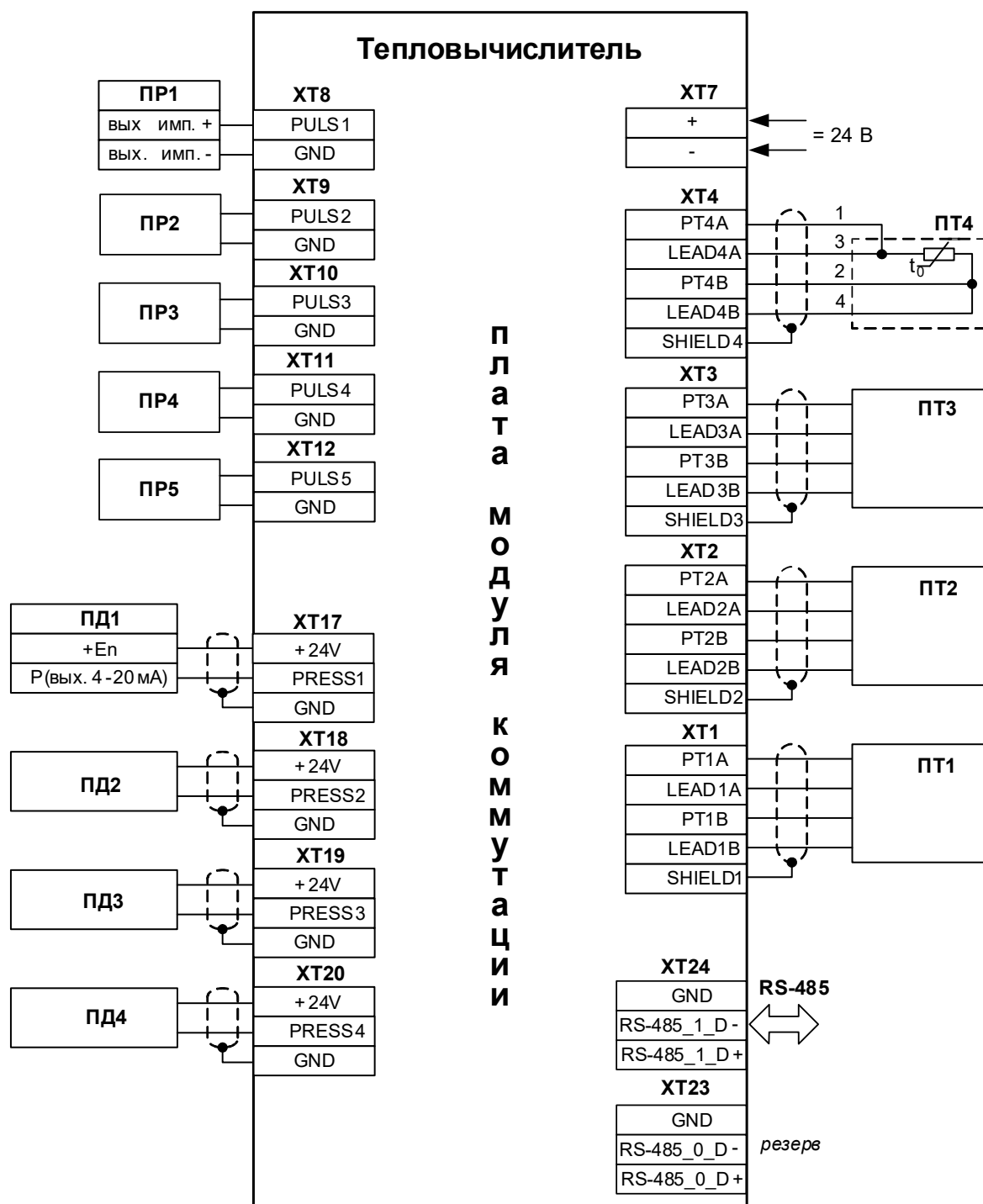
Рис.Б.1. Схема подключений к плате модуля коммутации.
