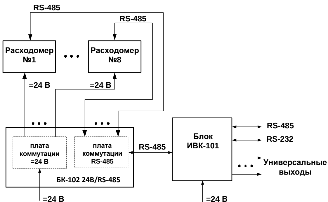
Рис.5. Система сбора данных и выносной индикации на базе комплекса «ВЗЛЕТ ИБК» исполнения ИБК-101 с использованием БК-102 для 2-8 расходомеров.
