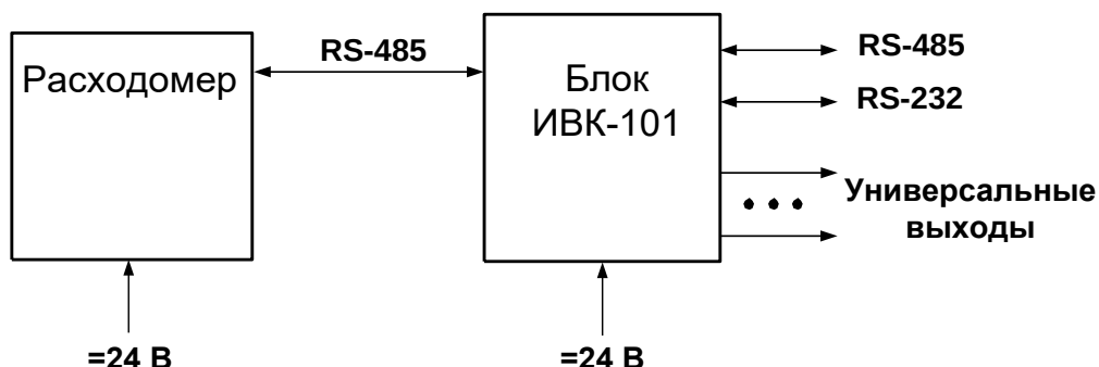
Рис.4. Система сбора данных и выносной индикации на базе комплекса «ВЗЛЕТ ИБК» исполнения ИБК-101 для одного расходомера.
