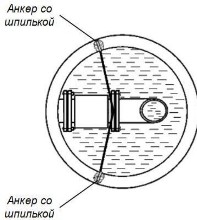
Рис.8. Монтаж расходомера в безнапорный трубопровод. Вид сверху.
