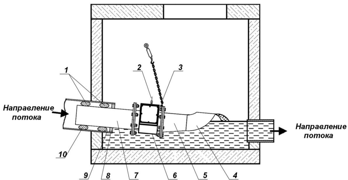
б) наклонное расположение расходомера
