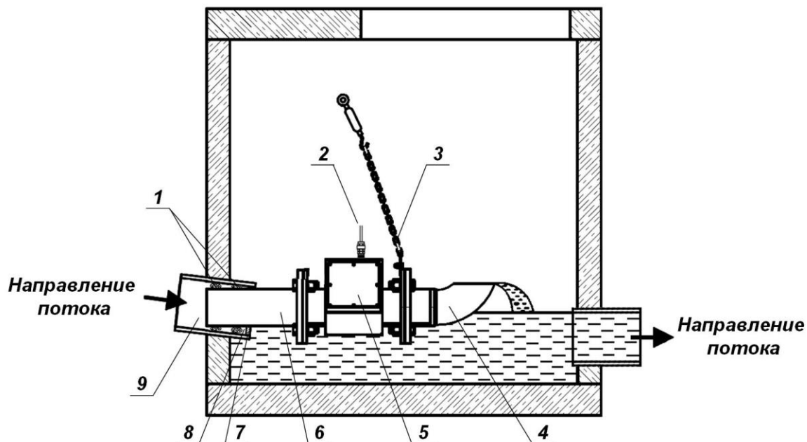
а) горизонтальное расположение расходомера
