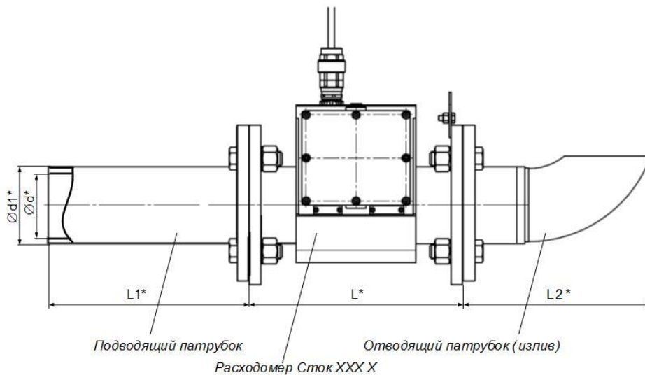
Рис.А.2. Сборная конструкция с подводящим патрубком и изливом для установки в безнапорные трубопроводы (КМЧ №1).
