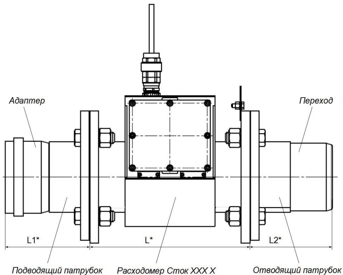
Рис.А.6. Сборная конструкция для установки в пластиковый трубопровод из труб НПВХ (КМЧ №4).
