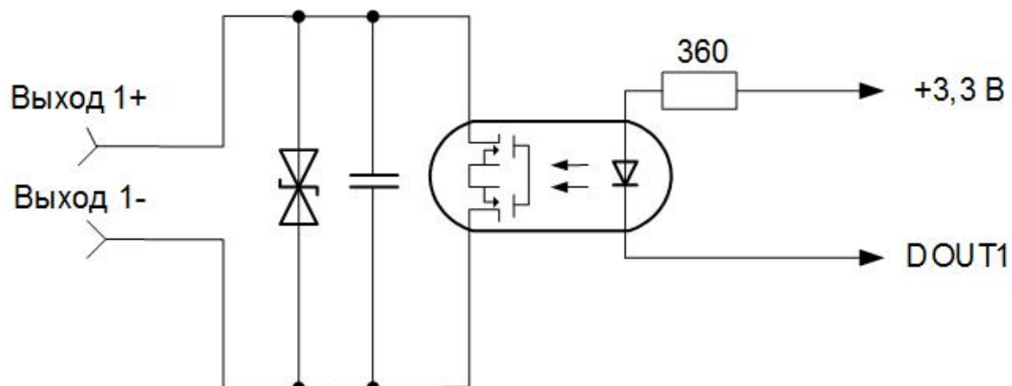
Рис.Б.1. Схема оконечного каскада универсальных выходов.
