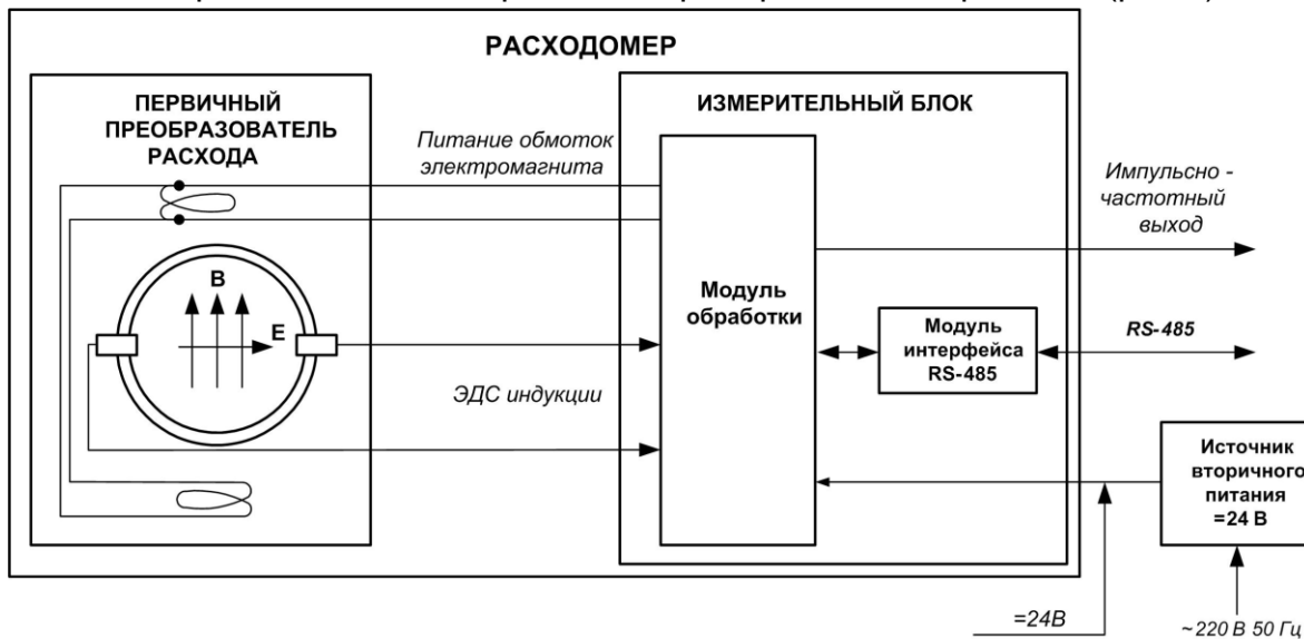
Рис.2. Структурная схема расходомера.
