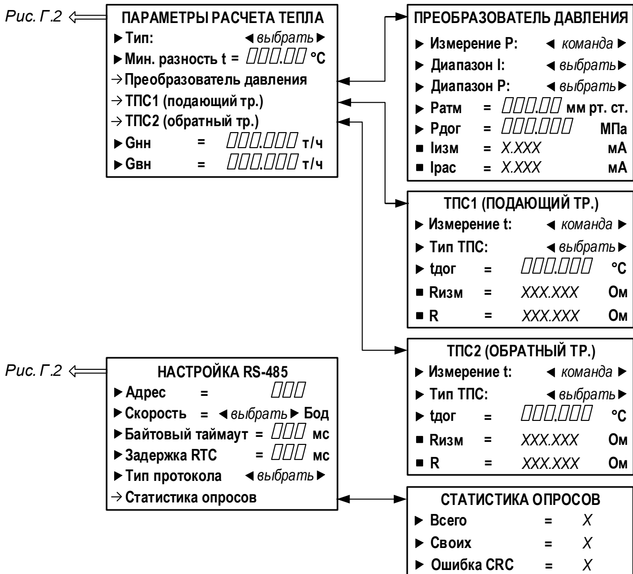
Рис.Г.5. Меню «ПАРАМЕТРЫ РАСЧЕТА ТЕПЛА» / «НАСТРОЙКА RS-485».
