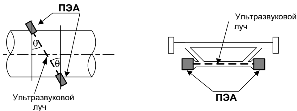
а) по диаметру либо по хорде б) в ИУ типа U-колена
