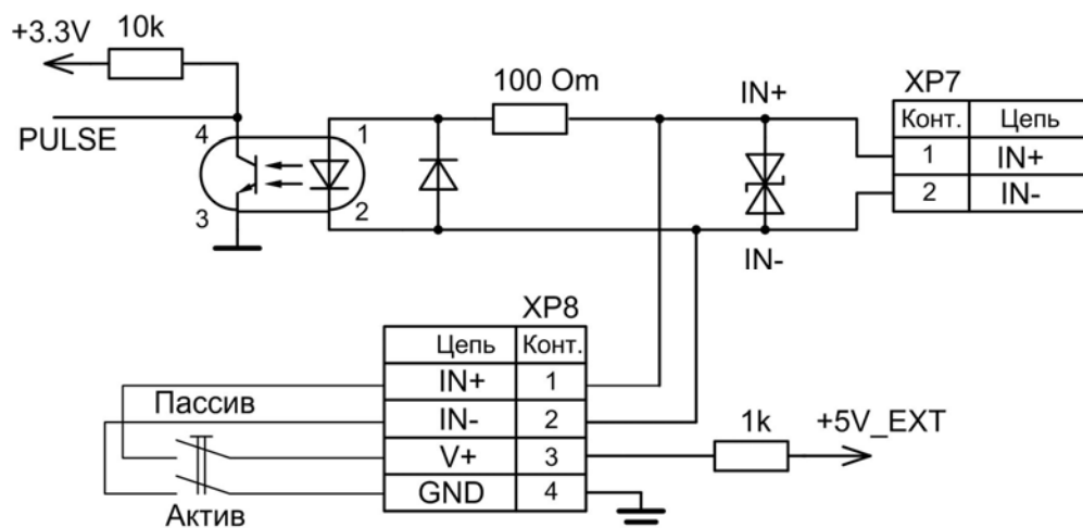
Рис. Б.1. Схема входного каскада частотно-импульсного входа
