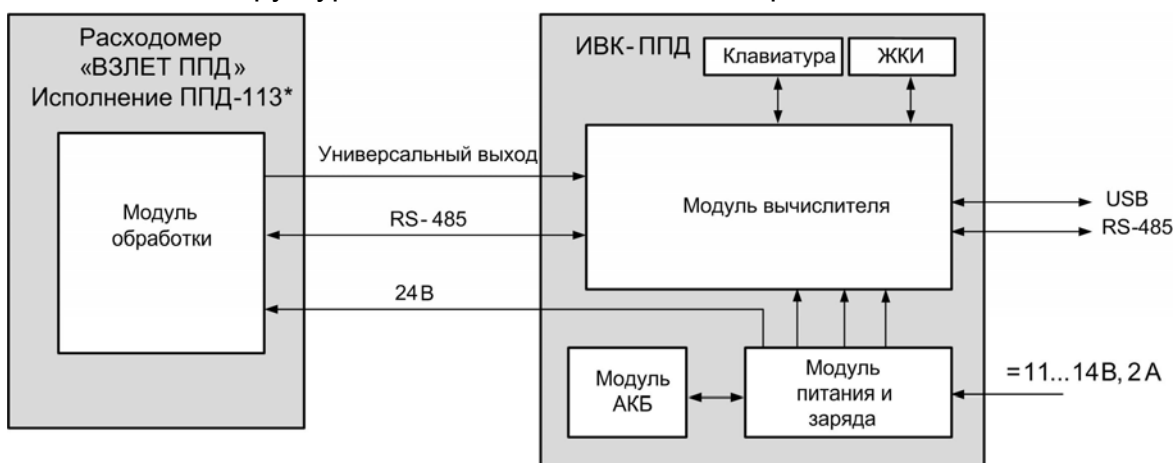
Рис. 1. Структурная схема ИВК-ППД.
