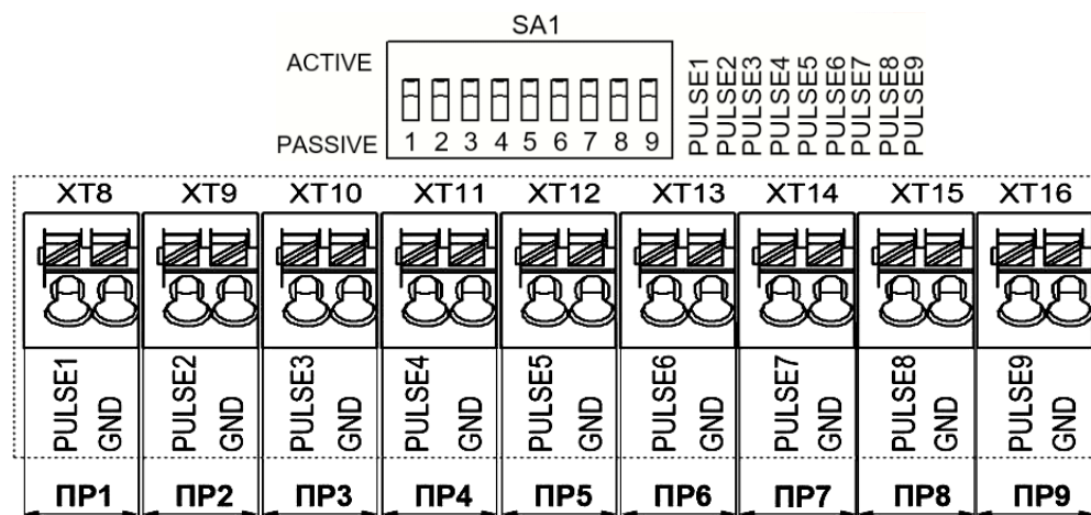
Рис.В.3. Коммутационные элементы подключения ПР1...ПР9.
