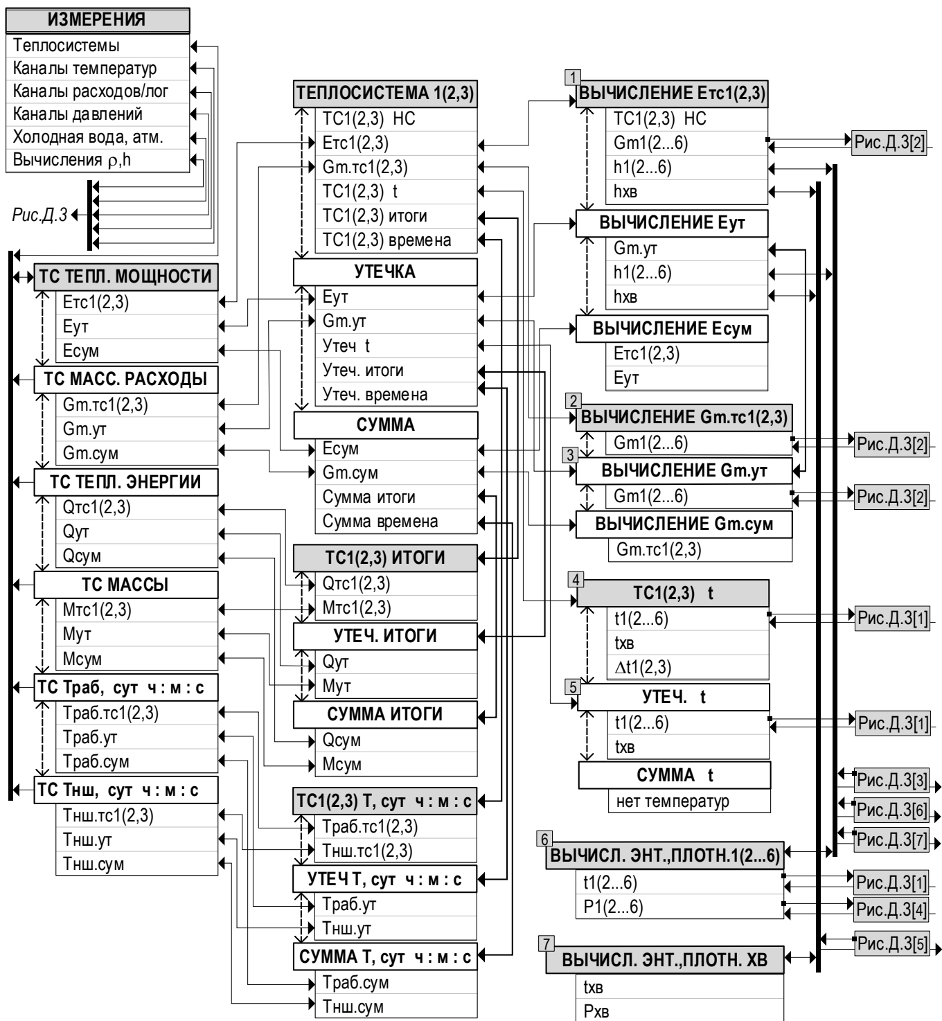
Рис.Д.2. Схема навигации в меню «Измерения» → «Теплосистемы» (режим РАБОТА).
