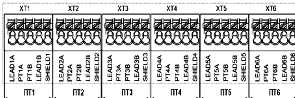
Рис.В.1. Коммутационные элементы подключения ПТ1...ПТ6.
