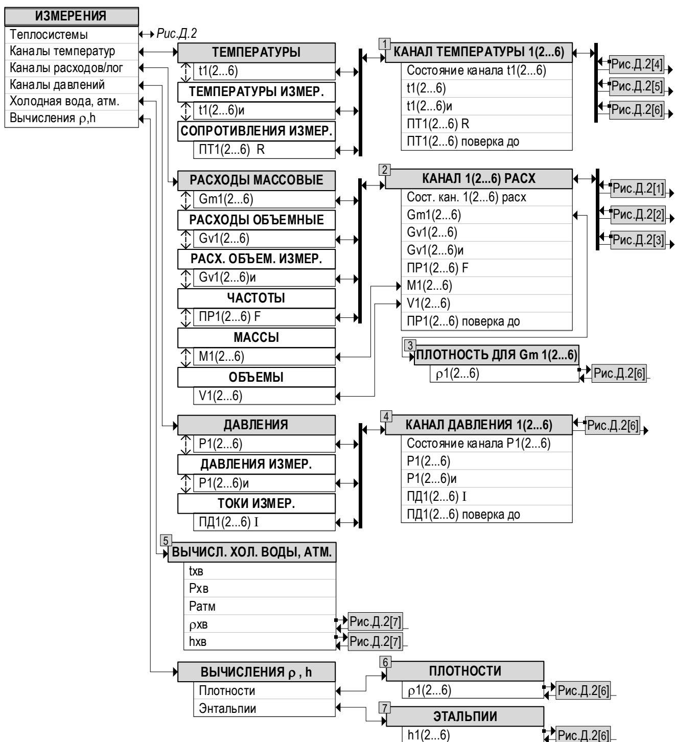
Рис.Д.3. Схема навигации в меню «Измерения»→ «Каналы температур», «Каналы расходов/лог», «Каналы давлений», «Холодная вода, атм.», «Вычисления ρ, h» (режим РАБОТА).
