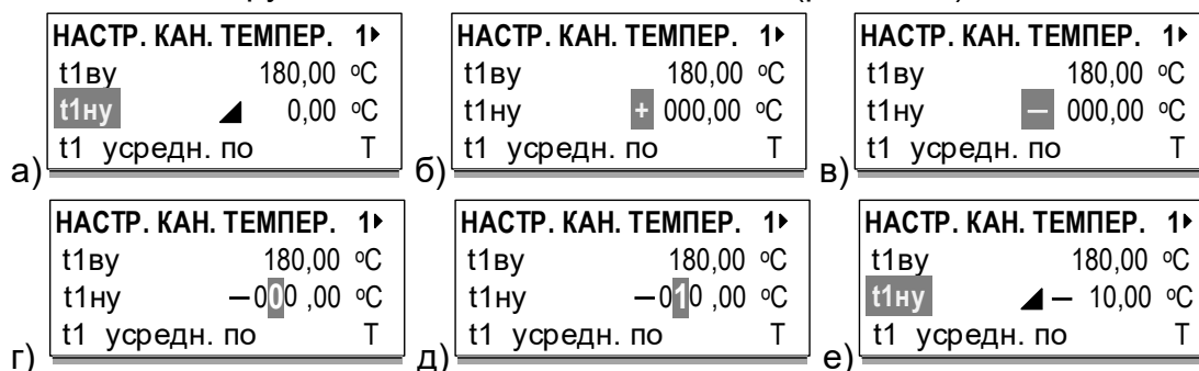
Рис.Б.3. Вид окна индикации при вводе значения параметра поразрядно.
