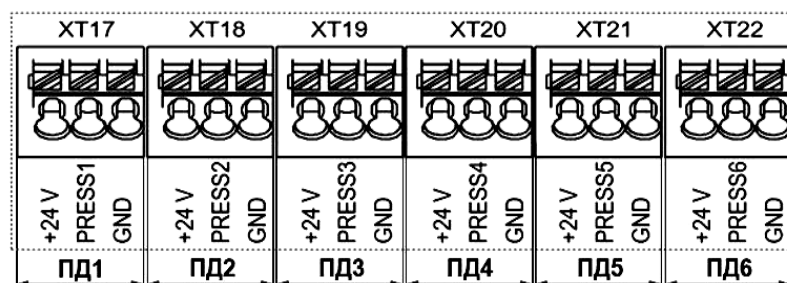
Рис.В.2. Коммутационные элементы подключения ПД1...ПД6.
