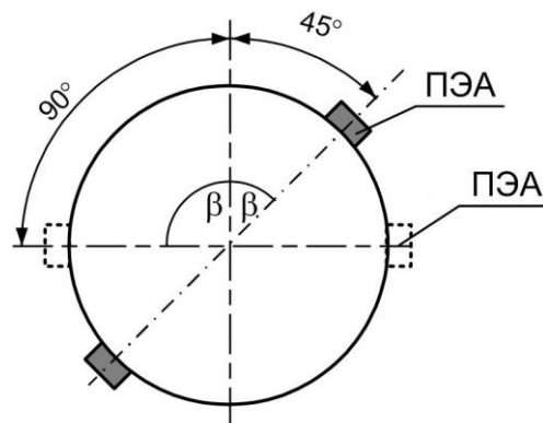
Рис.3. Рекомендуемое положение ПЭА на трубопроводе относительно вертикали.
