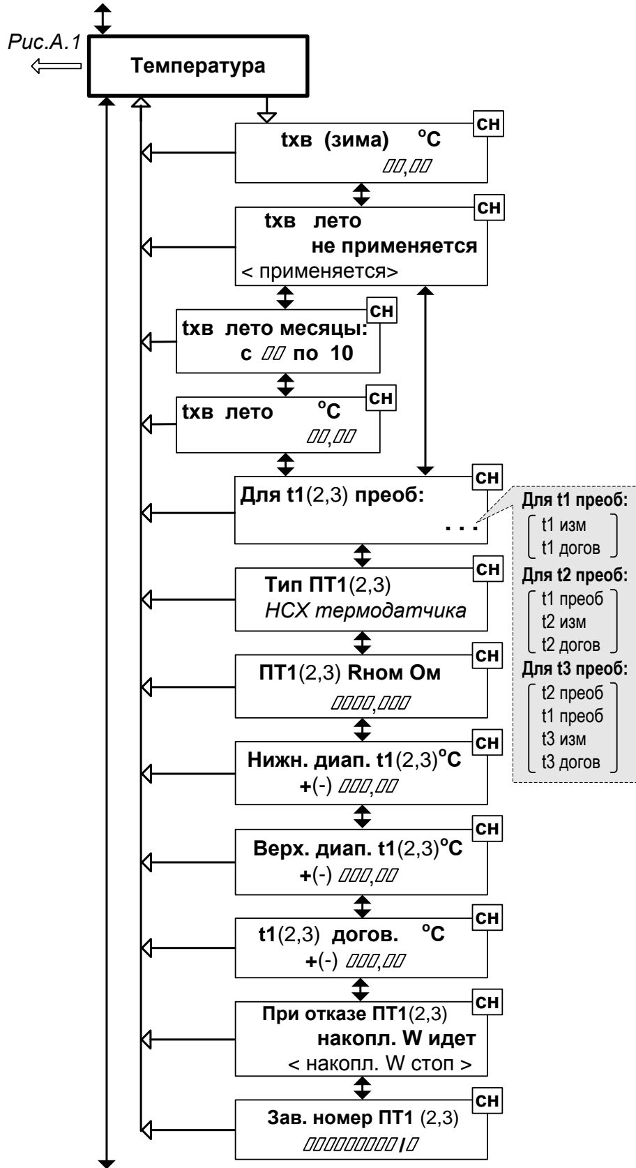
Рис.А.4. Состав и структура меню «УСТ / Температура».
