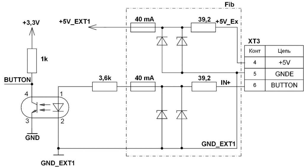
Рис.В.7 - Схема входного каскада входа управления
