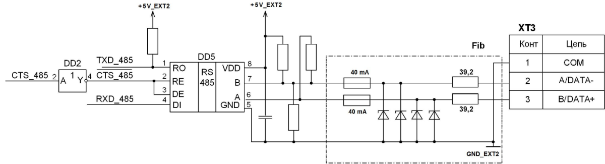
Рис.В.8 - Выход интерфейса RS-485.
