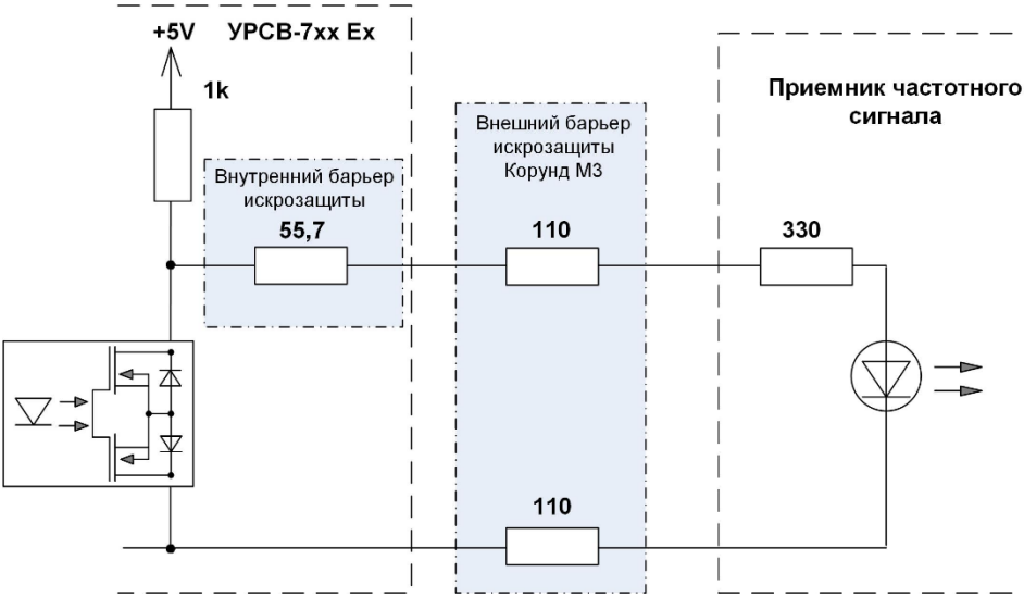
Рис.В.3 - Эквивалентная схема работы на низкоомную нагрузку.
