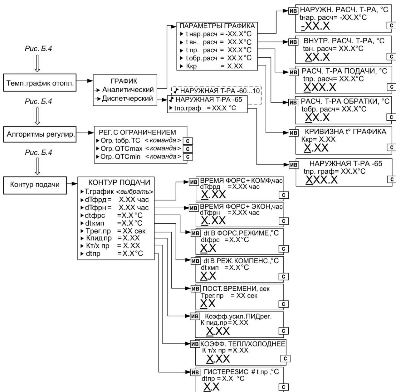
Рис.Б.4а. Вид меню «Температурный график отопления», «Алгоритмы регулирования» и «Контур подачи».
