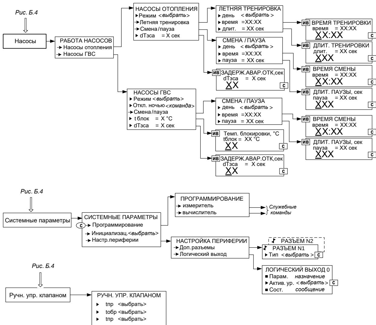
Рис.Б.4в. Вид меню «Насосы», «Системные параметры» и «Ручное управление клапаном».
