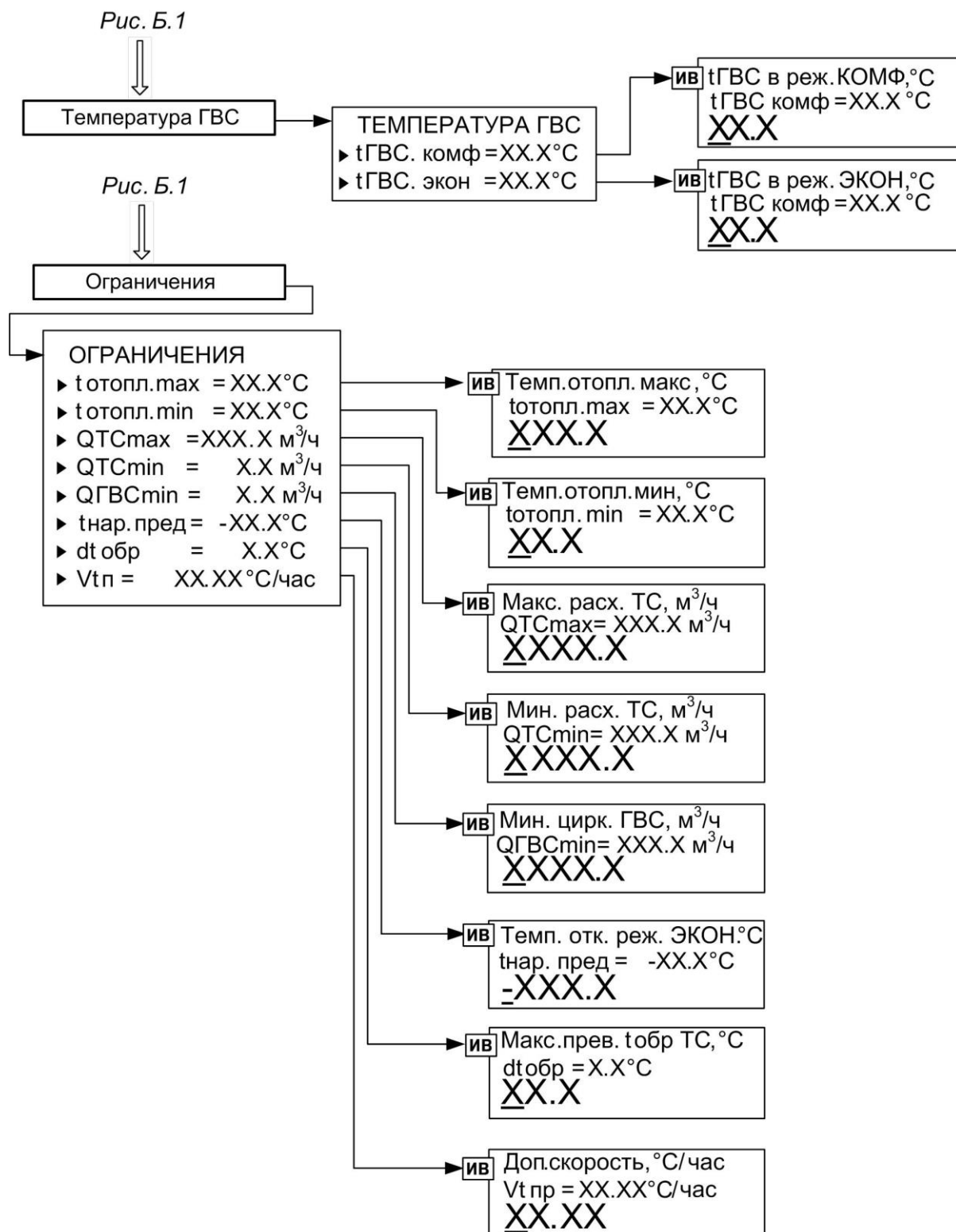
Рис.Б.2. Вид меню «Температура ГВС» и «Ограничения».
