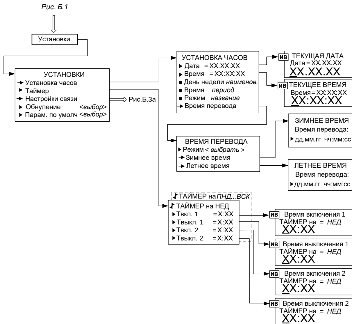
Рис.Б.3. Вид меню «Установки».
