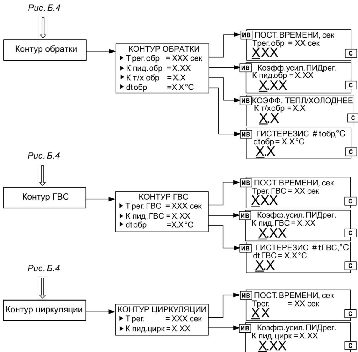
Рис.Б.4б. Вид меню «Контур обратной», «Контур ГВС» и «Контур циркуляции».
