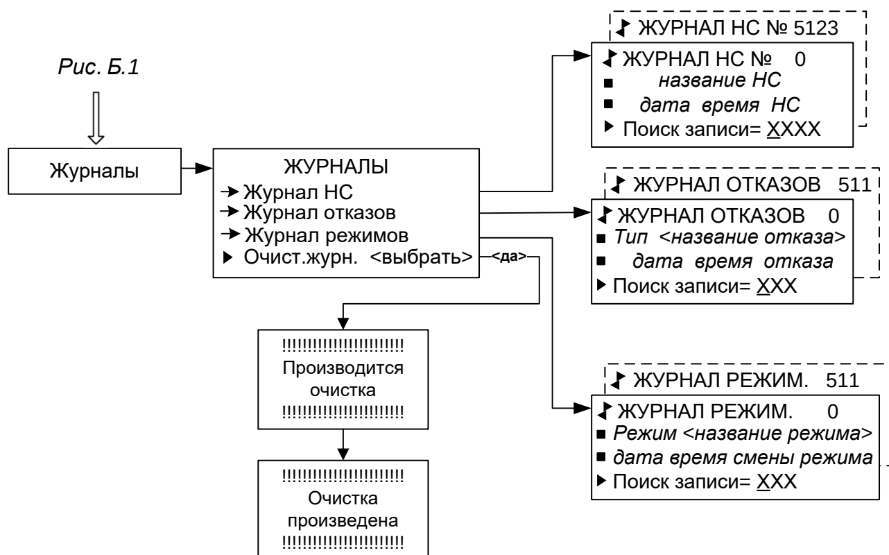
Рис.Б.7. Вид меню «Журналы».
