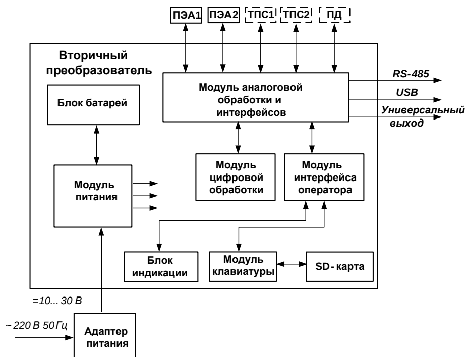
Рис.3. Структурная схема расходомера.
