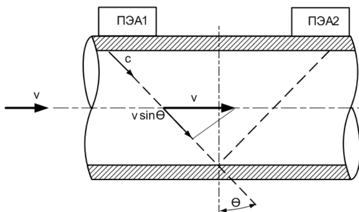
Рис.1. Схема прохождения УЗС.
