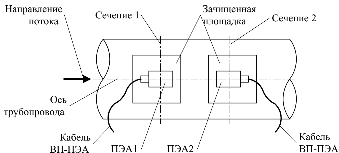
Рис. 8. Положение накладных ПЭА на трубопроводе.
