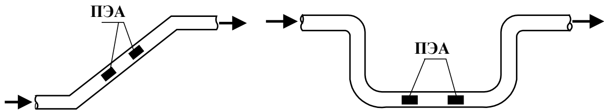
Рис. 1. Рекомендуемые места установки ПЭА (ПП).
