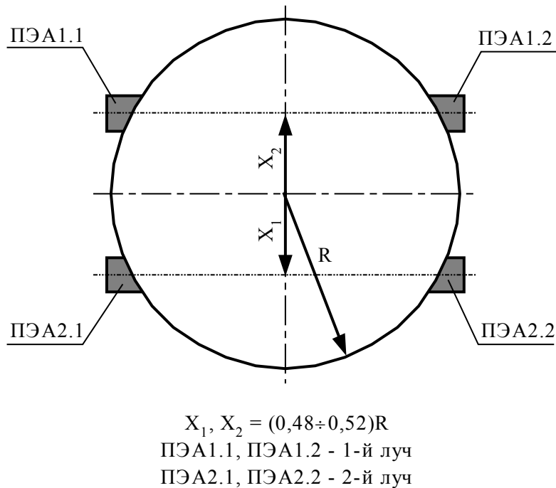
Рис. 3. Положение врезных ПЭА в проекции на перпендикулярное сечение трубопровода при типовом монтаже.
