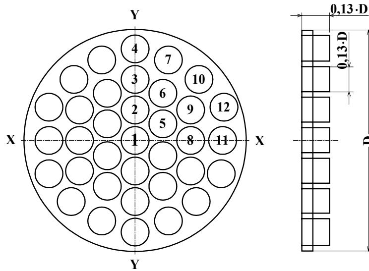
Рис. Л.2. Схема струевыпрямителя потока типа В.
