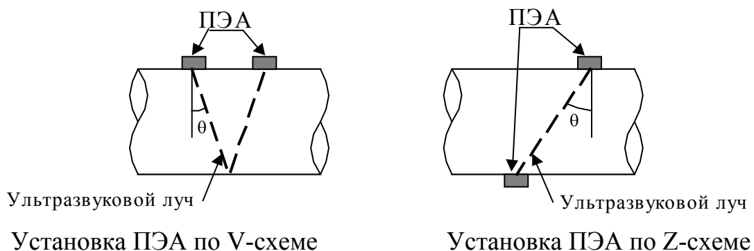
Рис. 2. Положение накладных ПЭА на трубопроводе.
