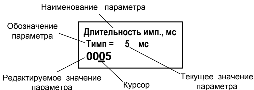
Рис.11. Вид окна индикации установочного параметра.
