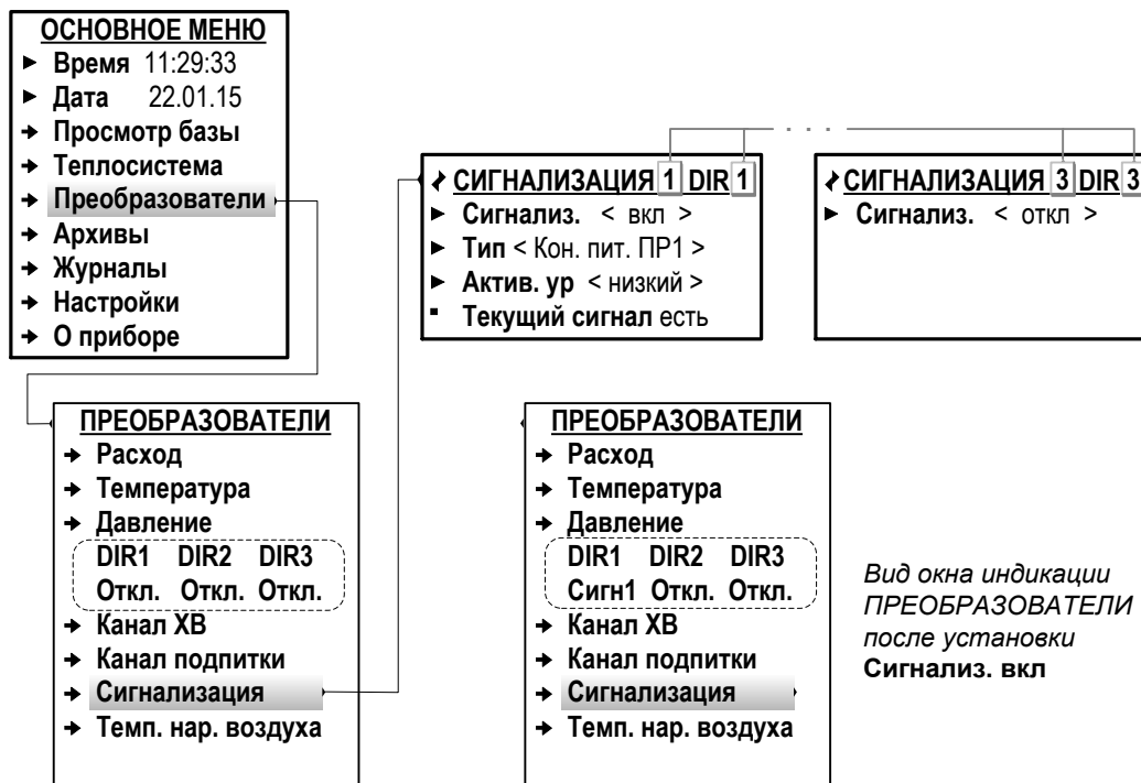
Рис.27. Вид меню настройки входов «Сигнализация» (режим СЕРВИС).
