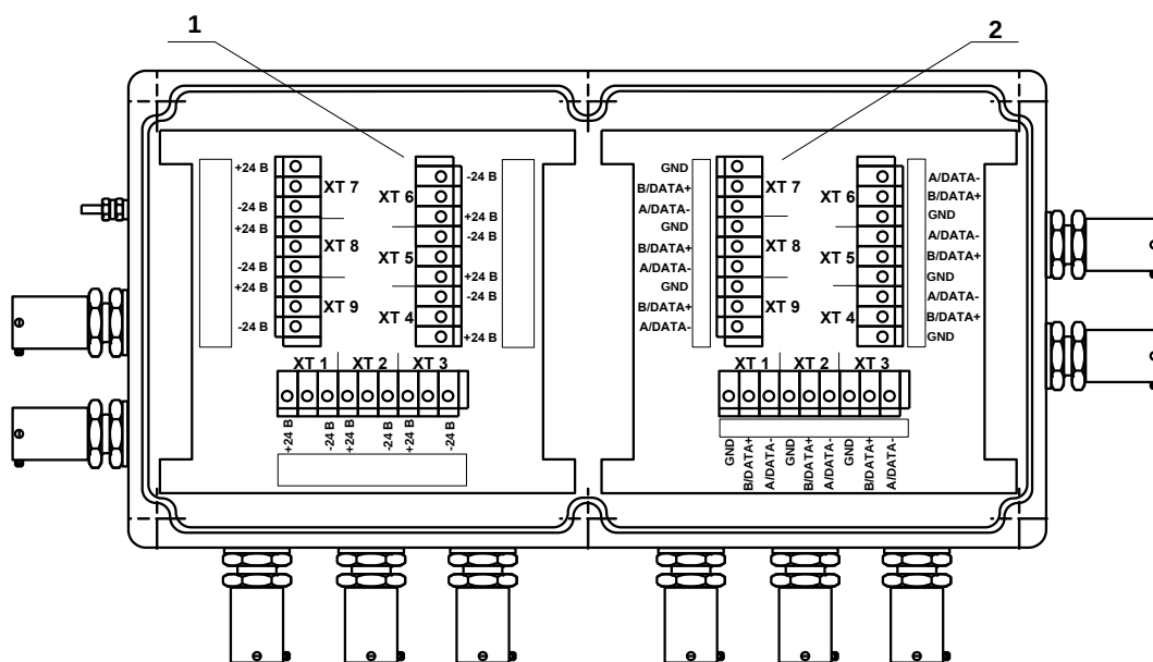
Рис.А.6. Блок коммутации БК-102 24B/RS-485.
