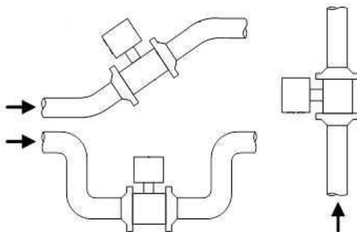
Рис.1. Рекомендуемые места установки расходомера.
