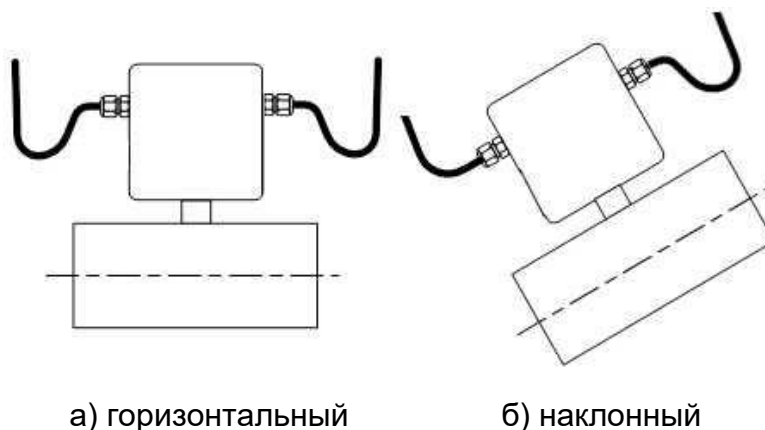
Рис.3. Положение кабелей на входе в гермовводы при монтаже ЭМР в трубопровод.
