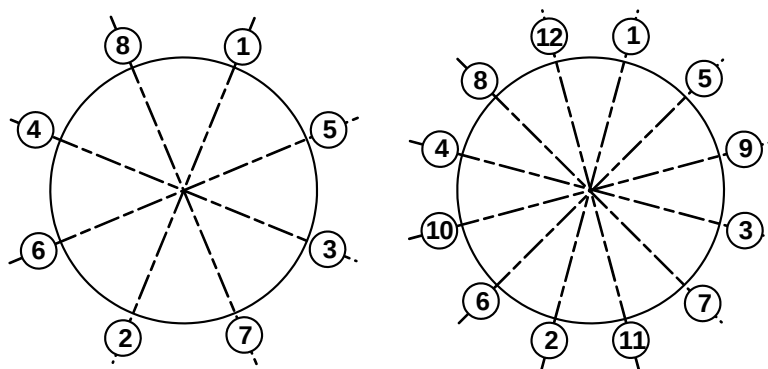
Рис.2. Очередность затяжки гаек на фланцах.
