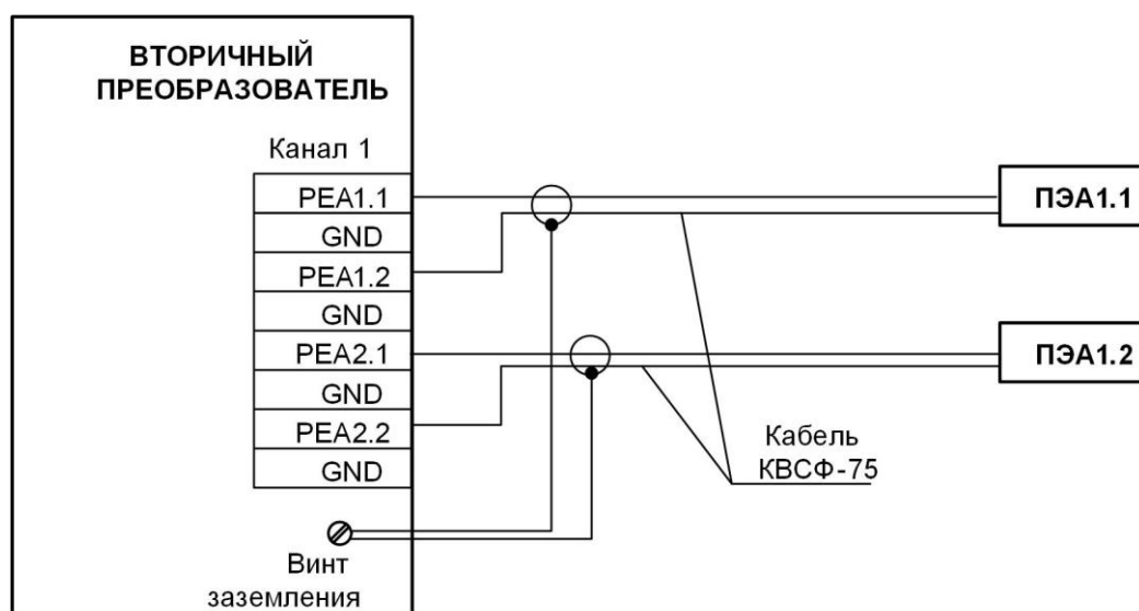
Рис.Б.2. Схема подключения ПЭА при использовании кабеля KVCF-75.
