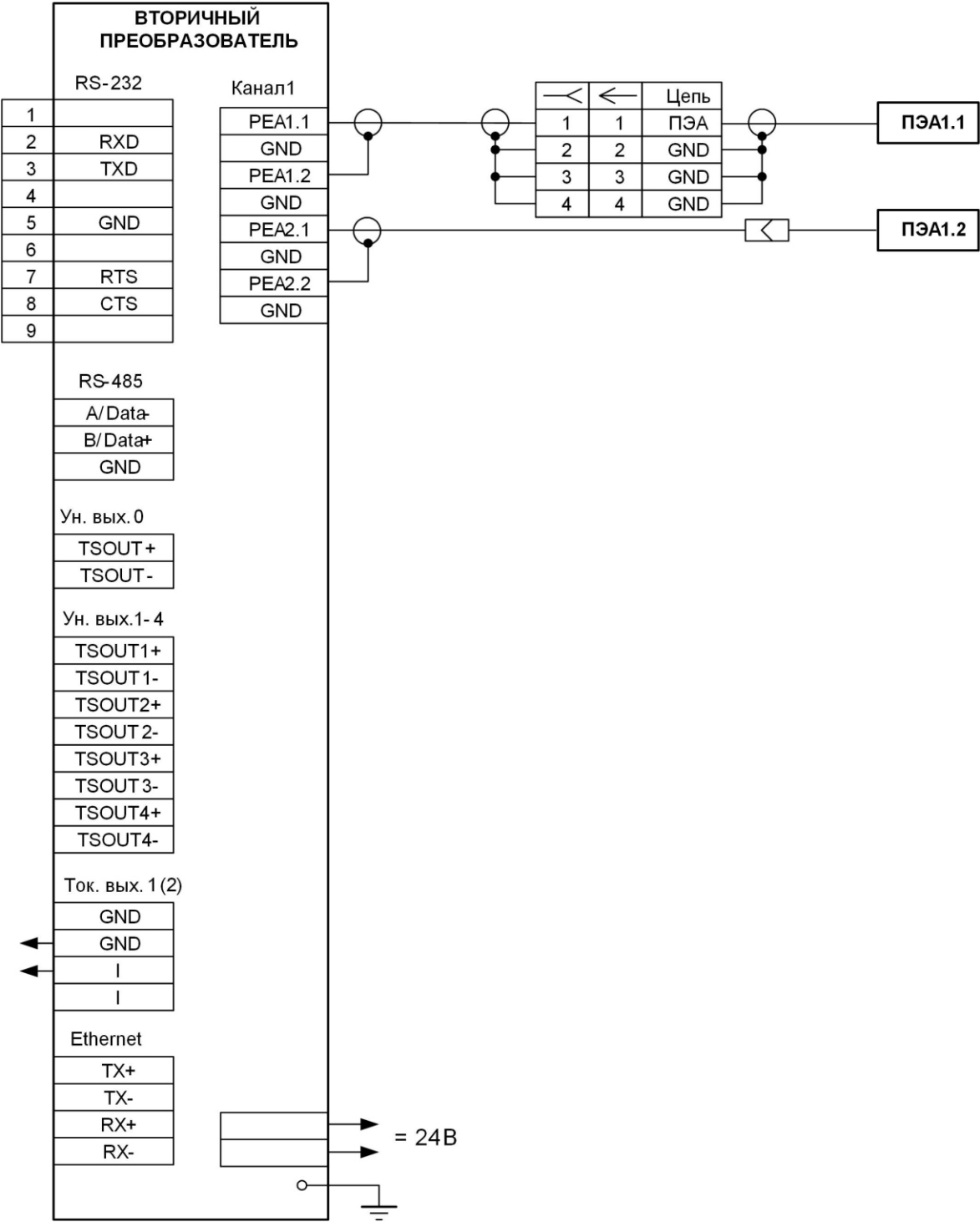
Рис.Б.1. Схема соединений расходомера исполнения УРСВ-510V.
