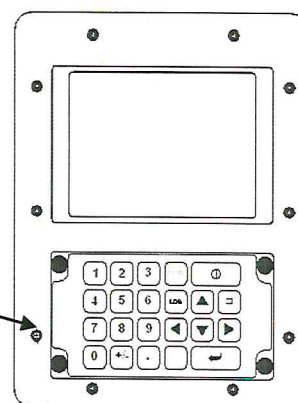
Рисунок 2 - Схема пломбировки расходомеров-счетчиков ультразвуковых переносных «ВЗЛЕТ ПРЦ»
