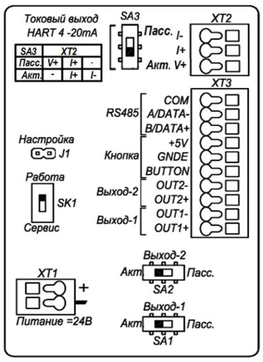
б) вид наклейки на задней крышке
