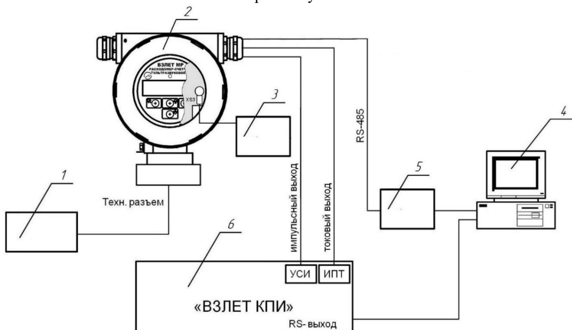
Рис.И.1 - Структурная схема поверки расходомера методом непосредственного сличения на поверочной установке.
