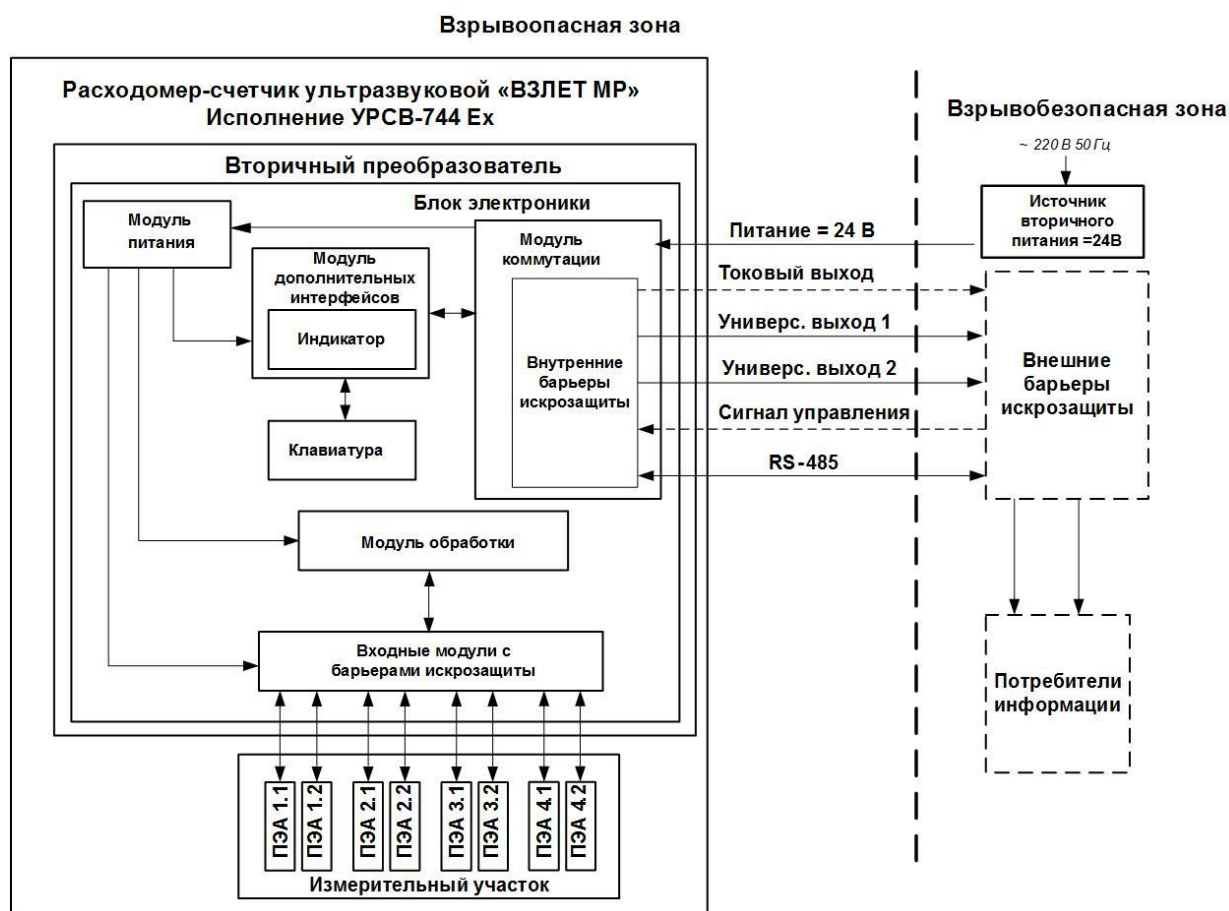
Рис.2 - Структурная схема четырехлучевого исполнения расходомера
