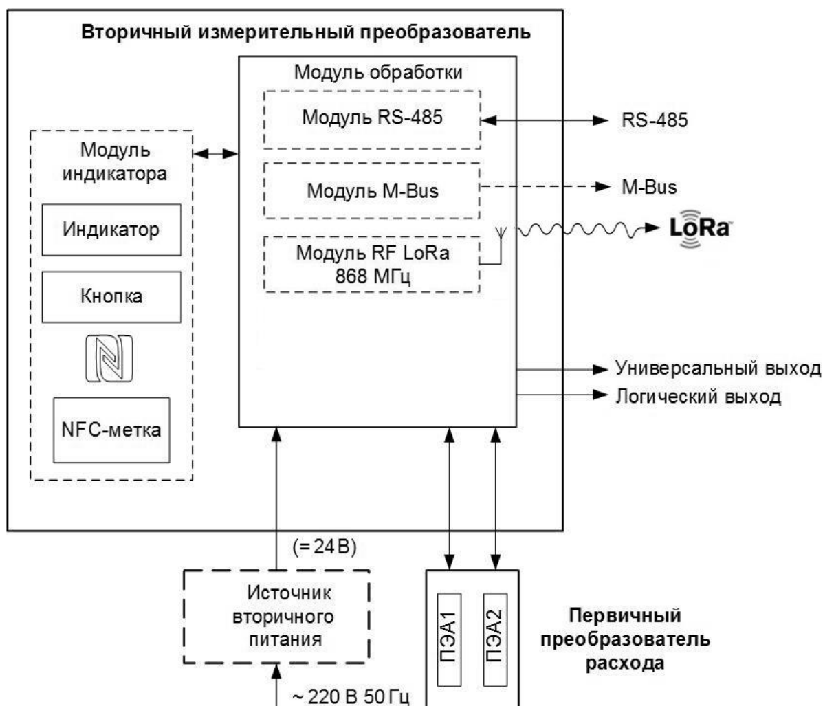
Рис.2. Структурная схема расходомера.
