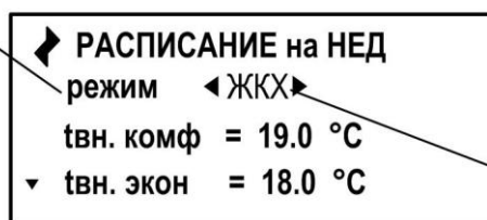
Рис.2. Пример установки режима отопления в меню «РАСПИСАНИЕ на НЕД».
