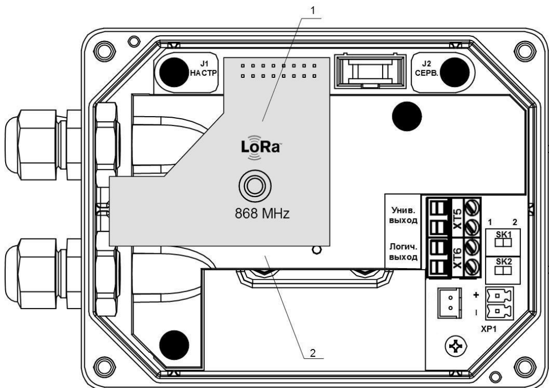
1 – модуль RF LoRa 868 МГц; 2 – экран.
